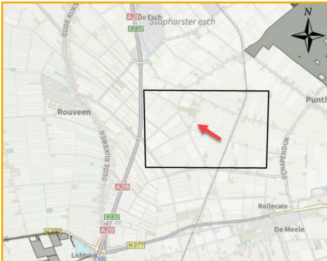
Figuur 4. Overzicht van plangebied (rode pijl) met ligging t.o.v. het NatuurNetwerk Nederland. (Bron: NDFF).
