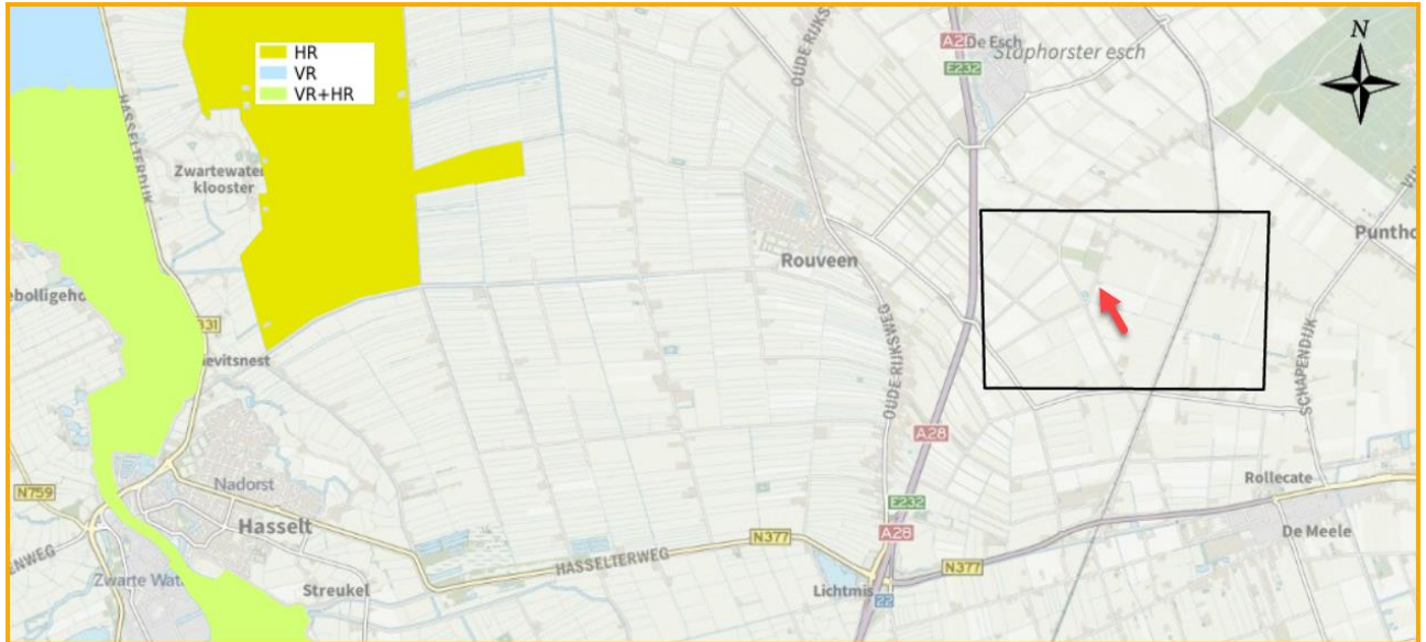
Figuur 5. Ligging van het plangebied (rode pijl) ten opzichte van Natura 2000-gebieden. (Bron: NDFF).
