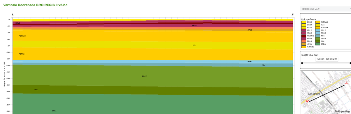
figuur 2: geohydrologische opbouw
