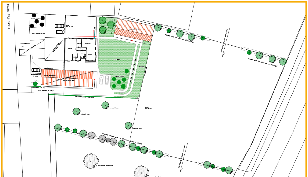
Figuur 2. Plantekening nieuwe situatie
