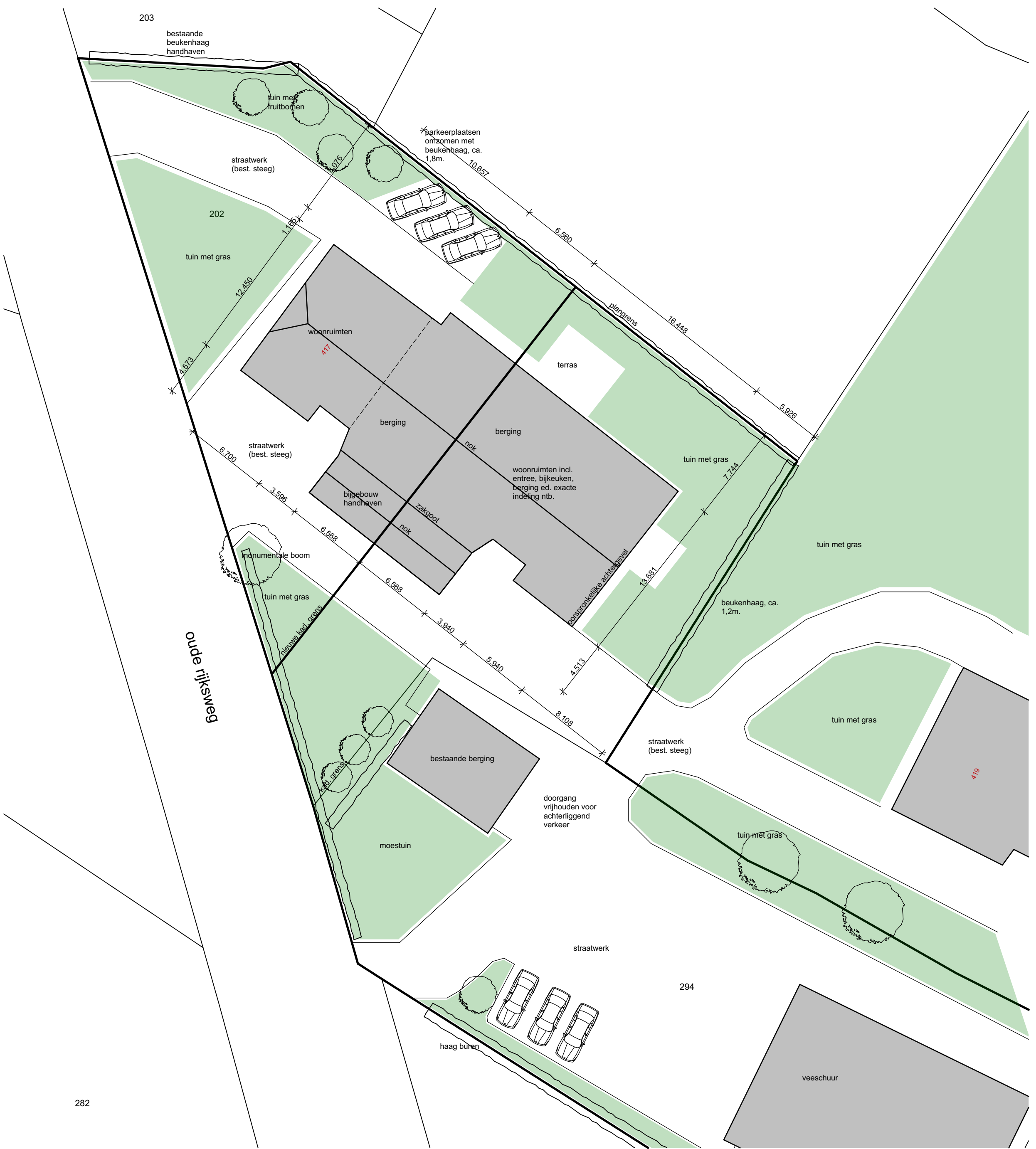
gewijzigde erfindingeling 1:250
