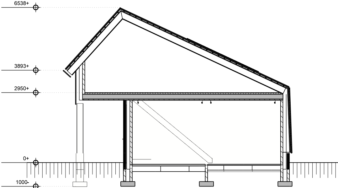
Doorsnede E-E
