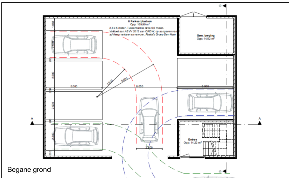
Afbeelding 2.4 Plattegrond begane grond (Bron: Bouwbureau Jansman)
