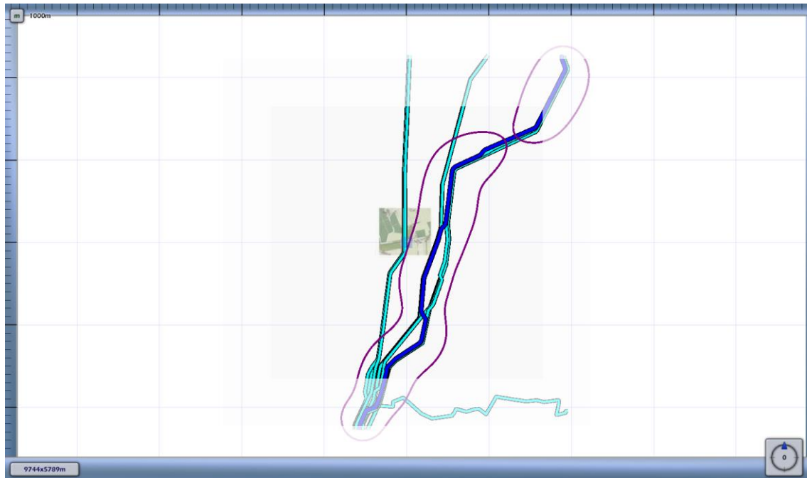
k. Figuur 3.11 Plaatsgebonden risico voor 7553_leiding-A-661-deel-1 van N.V. Nederlandse Gasunie
