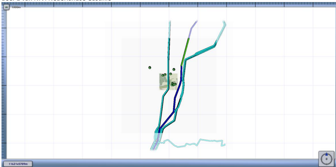
Figuur 4.5 Kilometer leiding behorende bij de maximale overschrijding van de FN-curve voor 7553_leiding-A-509-deel-1 van N.V. Nederlandse Gasunie
