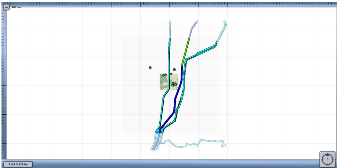
d. Figuur 4.4 Groepsrisico screening voor 7553_leiding-A-508-08-deel-1 van N.V. Nederlandse Gasunie
