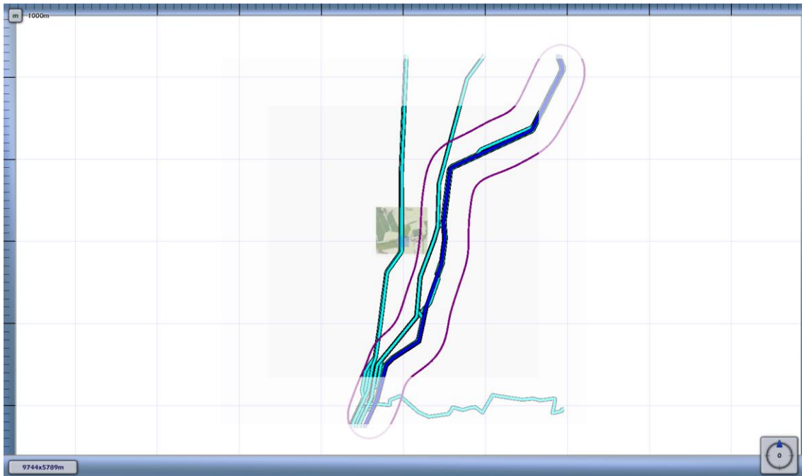
h. Figuur 3.8 Plaatsgebonden risico voor 7553_leiding-A-519-deel-1 van N.V. Nederlandse Gasunie
