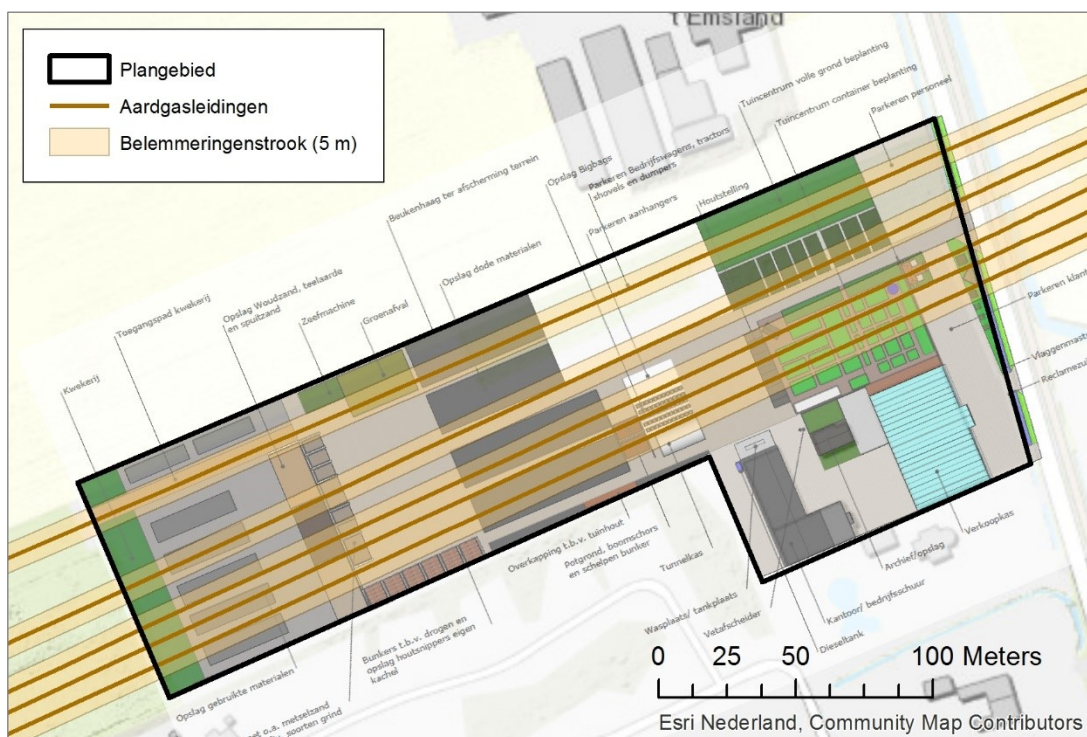
Figuur 2. Belemmeringenstroken rond aardgasleidingen
