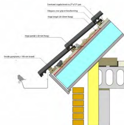
Grippaas in het dakvoetdetail
