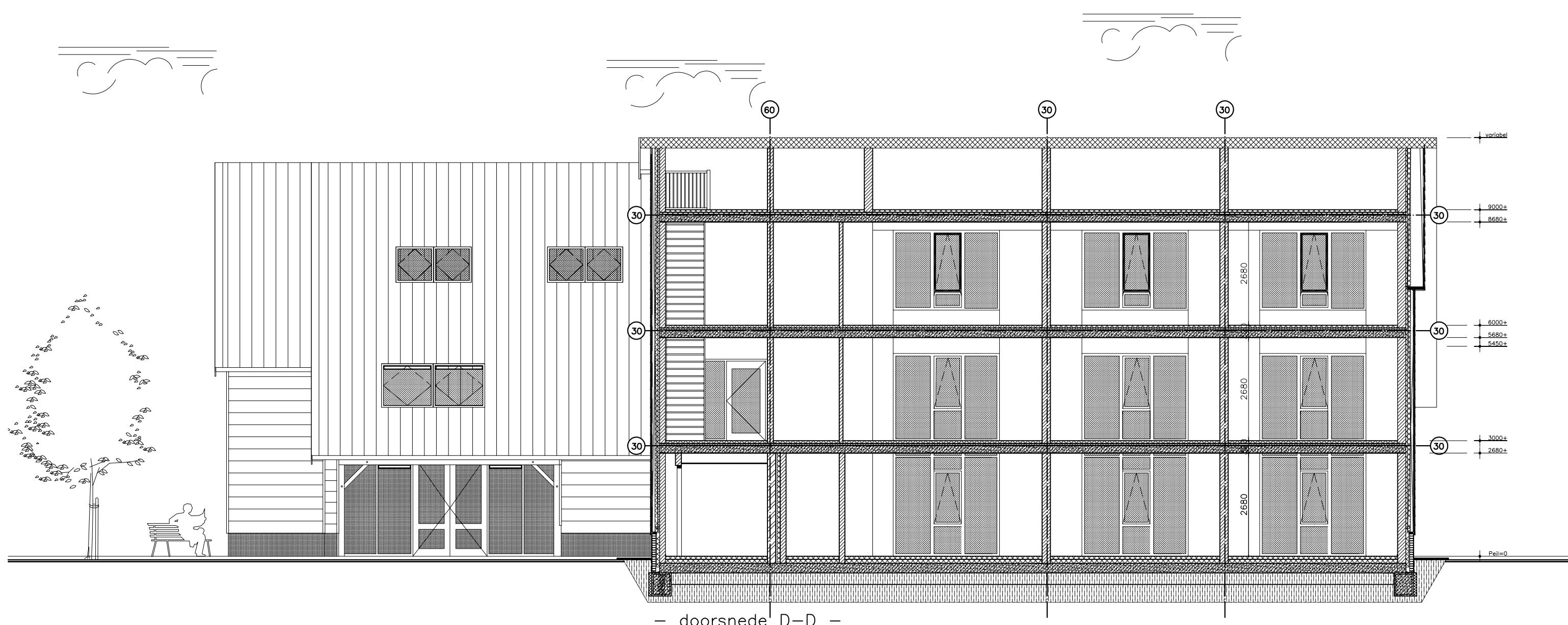
– doorsnede D-D –
