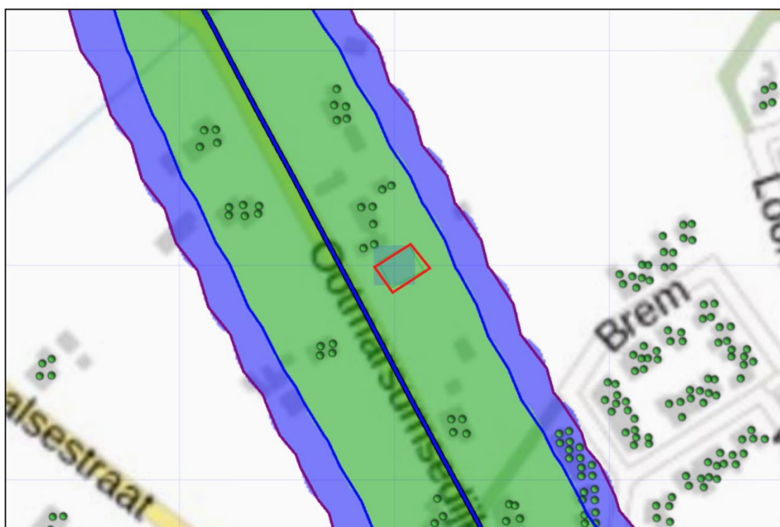
Figuur 3.1 Plaatsgebonden risico voor 7281_leiding-N-528-21-deel-1 van N.V. Nederlandse Gasunie
