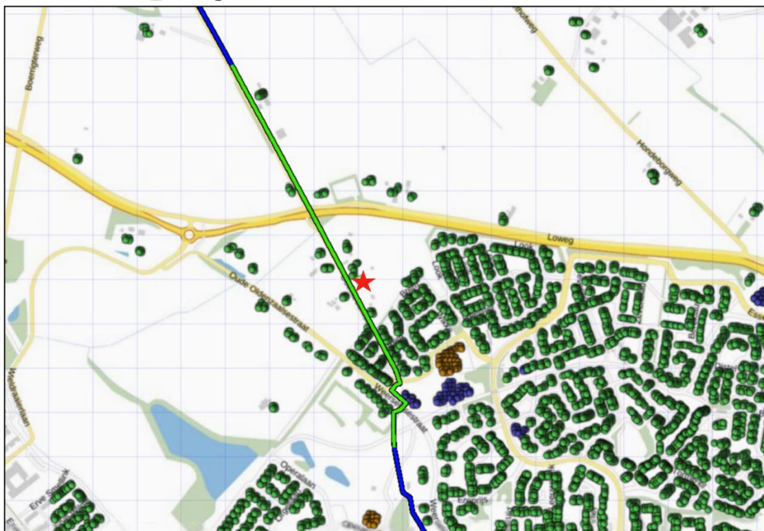
Figuur 4.2 Kilometer leiding behorende bij de maximale overschrijding van de FN-curve voor 7281_leiding-N-528-21-deel-1 van N.V. Nederlandse Gasunie
