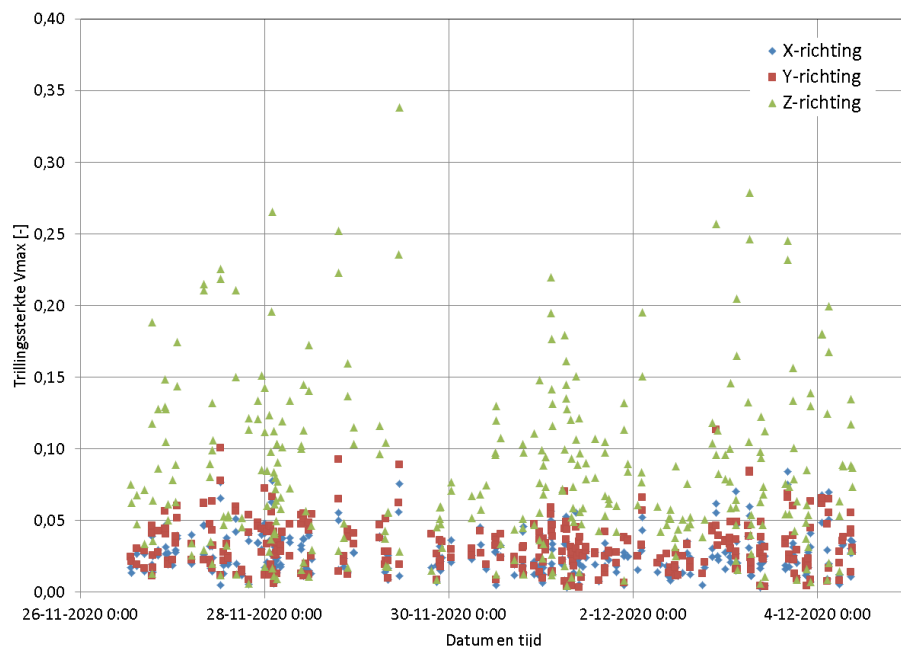
f2.3 Optredende maximale trillingssterkte in de bodem (meetlocatie 2)
