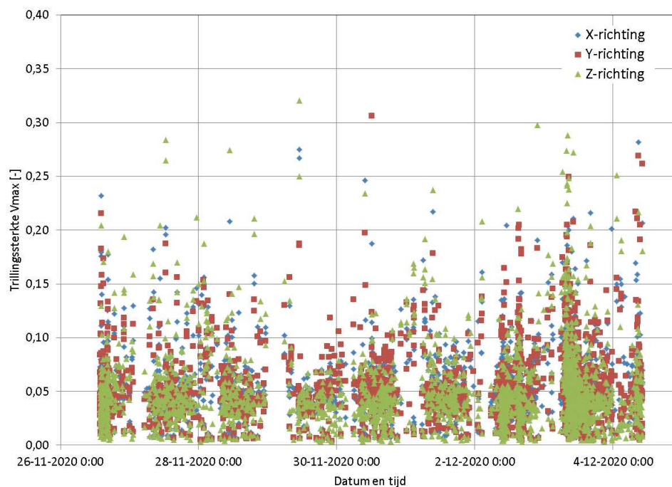
f2.2 Optredende maximale trillingssterkte in de bodem (meetlocatie 1)
