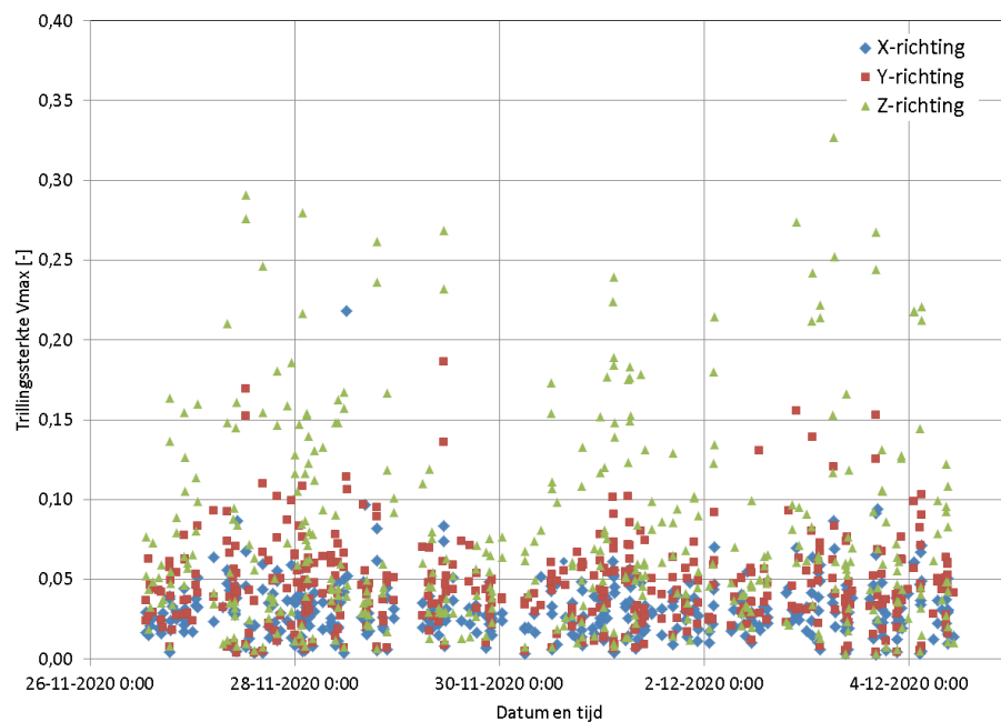
f2.4 Optredende maximale trillingssterkte in de bodem (meetlocatie 3)
