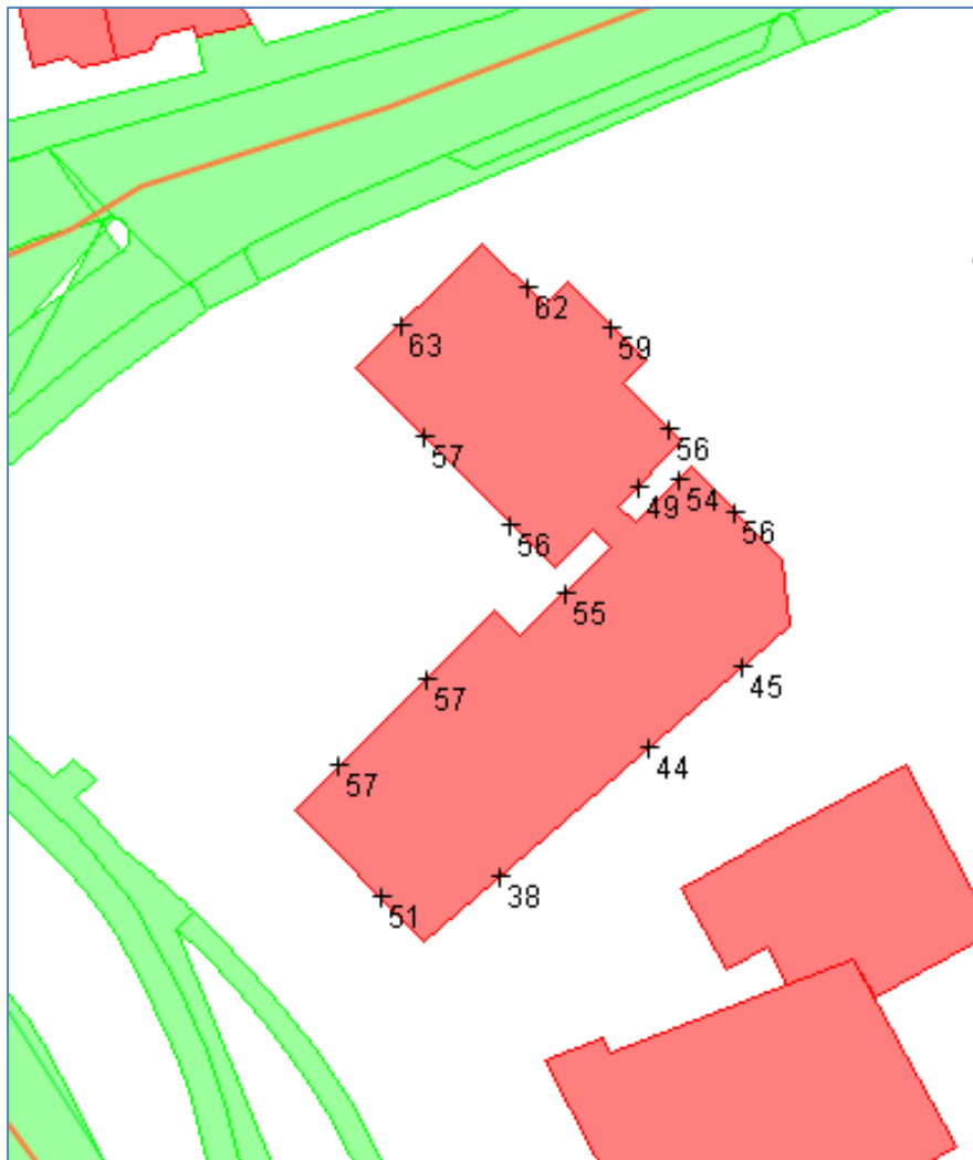
Figuur 3 Hoogst berekende geluidbelasting vanwege de Prins Bernhardstraat inclusief aftrek conform artikel 110 g Wgh
