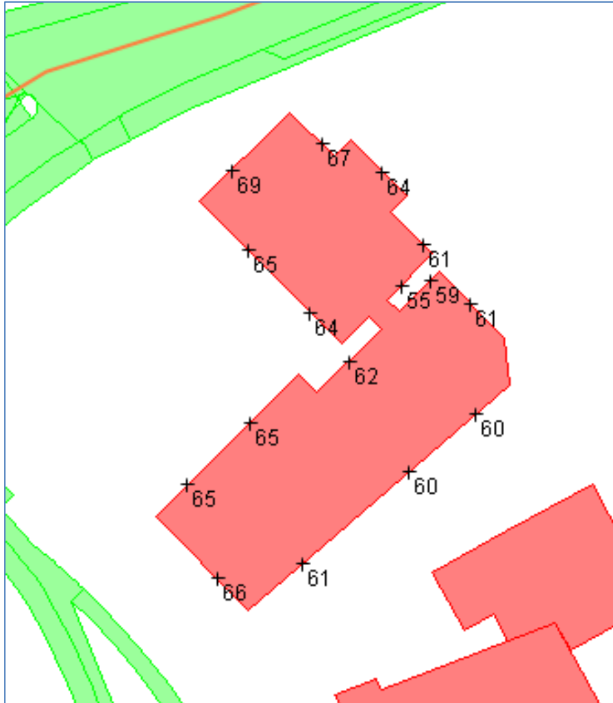
Figuur 5 Hoogst berekende geluidbelasting vanwege het gecumuleerd geluid exclusief aftrek conform artikel 110 g Wgh
