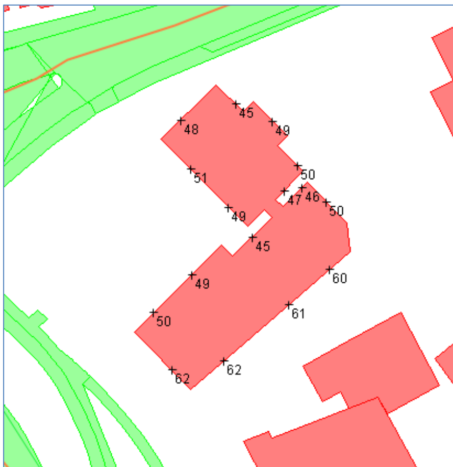
Figuur 4 Hoogst berekende geluidbelasting vanwege de Spoorlijn Oldenzaal-Hengelo
