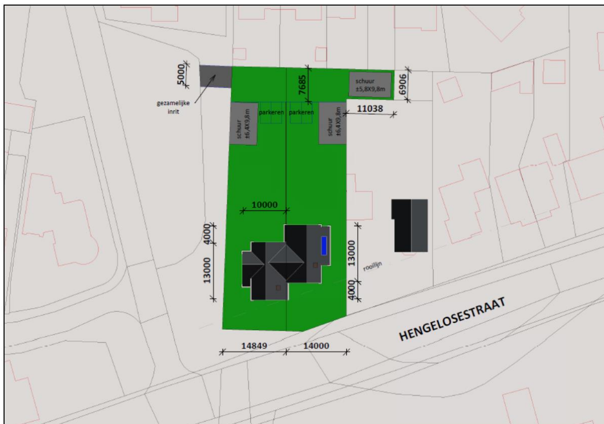
Afbeelding 3.1 Plattegrond gewenste situatie (Bron: Lassche Bouwregisseurs)
