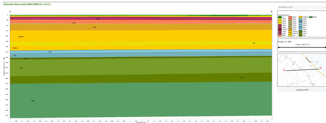
figuur 6: bodemopbouw
