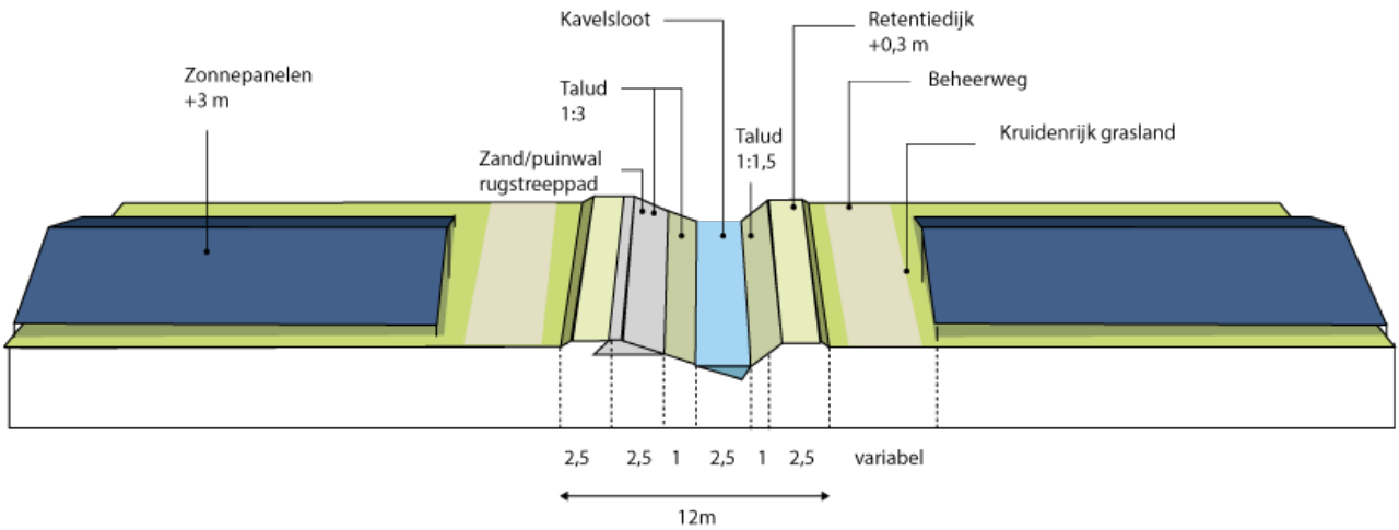
D. Principeprofiel zuidelijke kavelsloot: hier zou een zand/puinwal kunnen worden aangelegd ten behoeve van de rugstreppad
