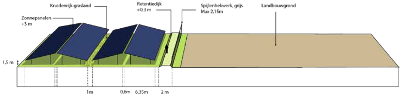
B. Principeprofiel rand zonneweide
