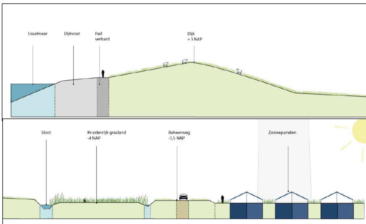
Profiel vanaf dijk (boven) naar zonneweide (onder).
