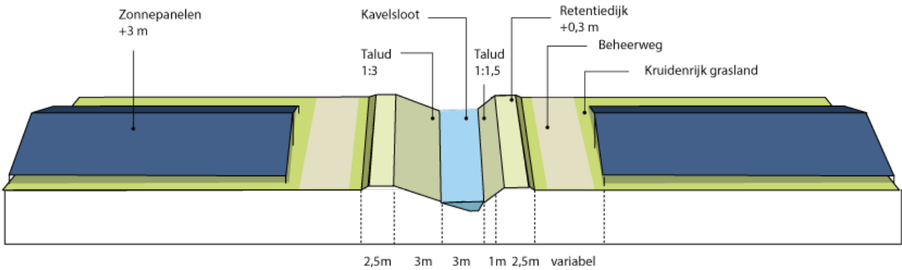
C. Principeprofiel kavelsloten
