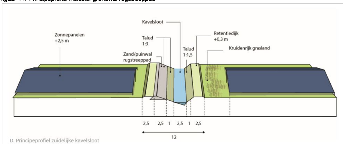
figuur 14. Principeprofiel inclusief grondwal rugstreeppad
