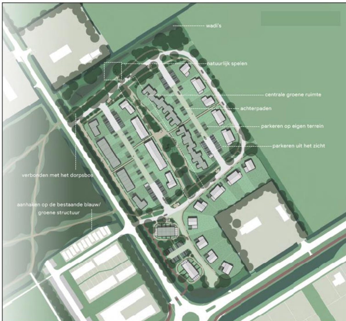
Afbeelding 2.1 Te realiseren situatie (Bron: Atelier Dutch)
