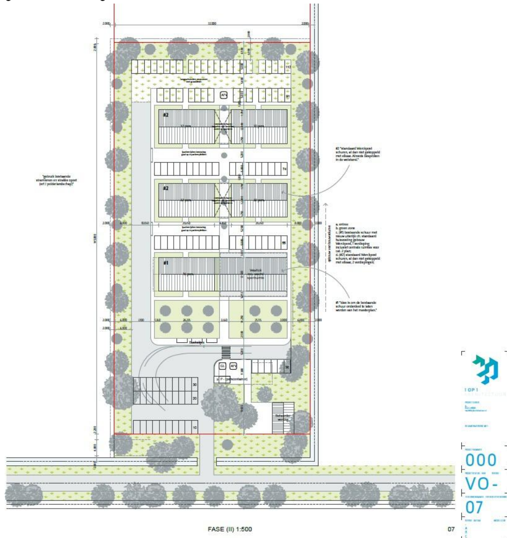
Afbeelding 17: Bouwtekening.
