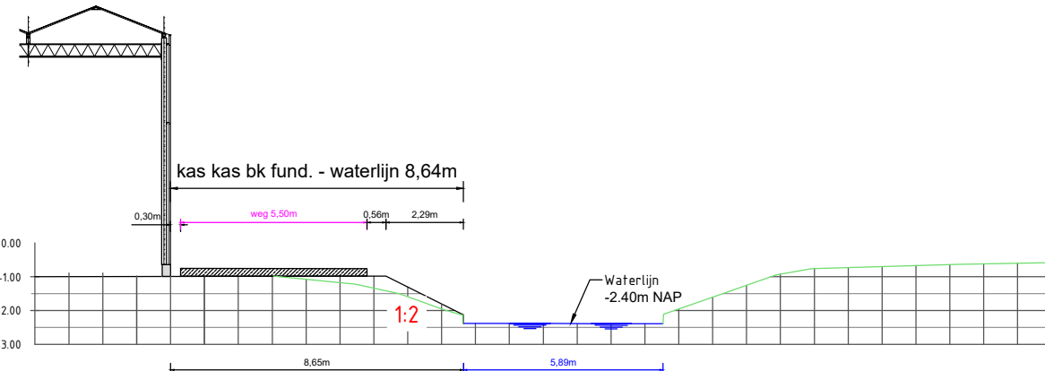
DWARSPROFIEL 2 Schaal 1:200
