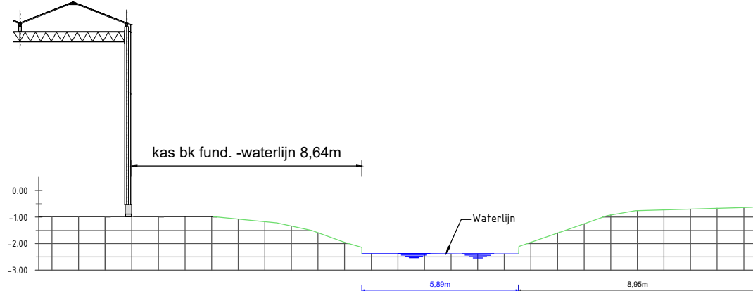
DWARSPROFIEL 2 Schaal 1:200
