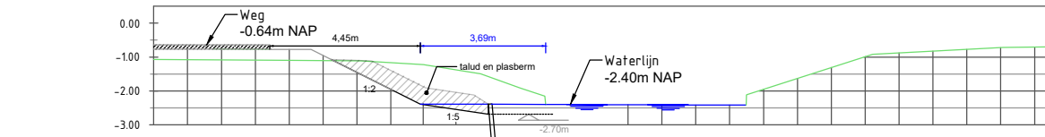
DWARSPROFIEL 1 Schaal 1:200
