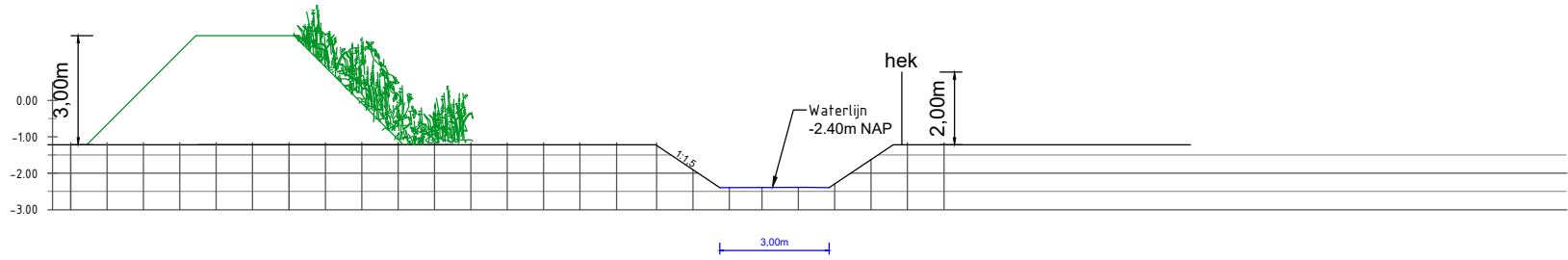
DWARSPROFIEL 4 Schaal 1:200
