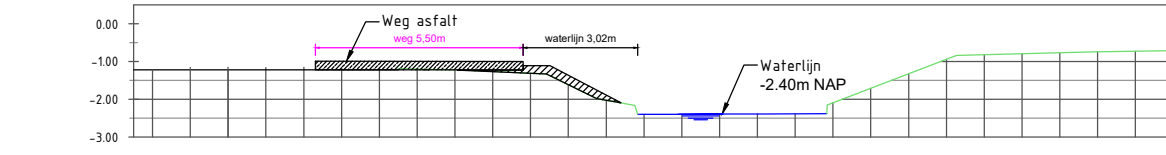
DWARSPROFIEL 3 Schaal 1:200
