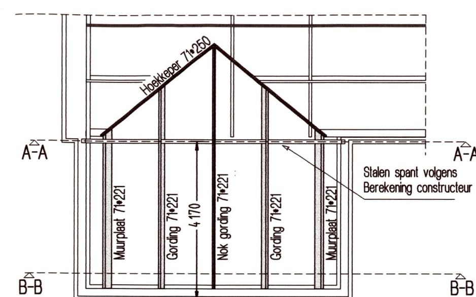
Kapplan
