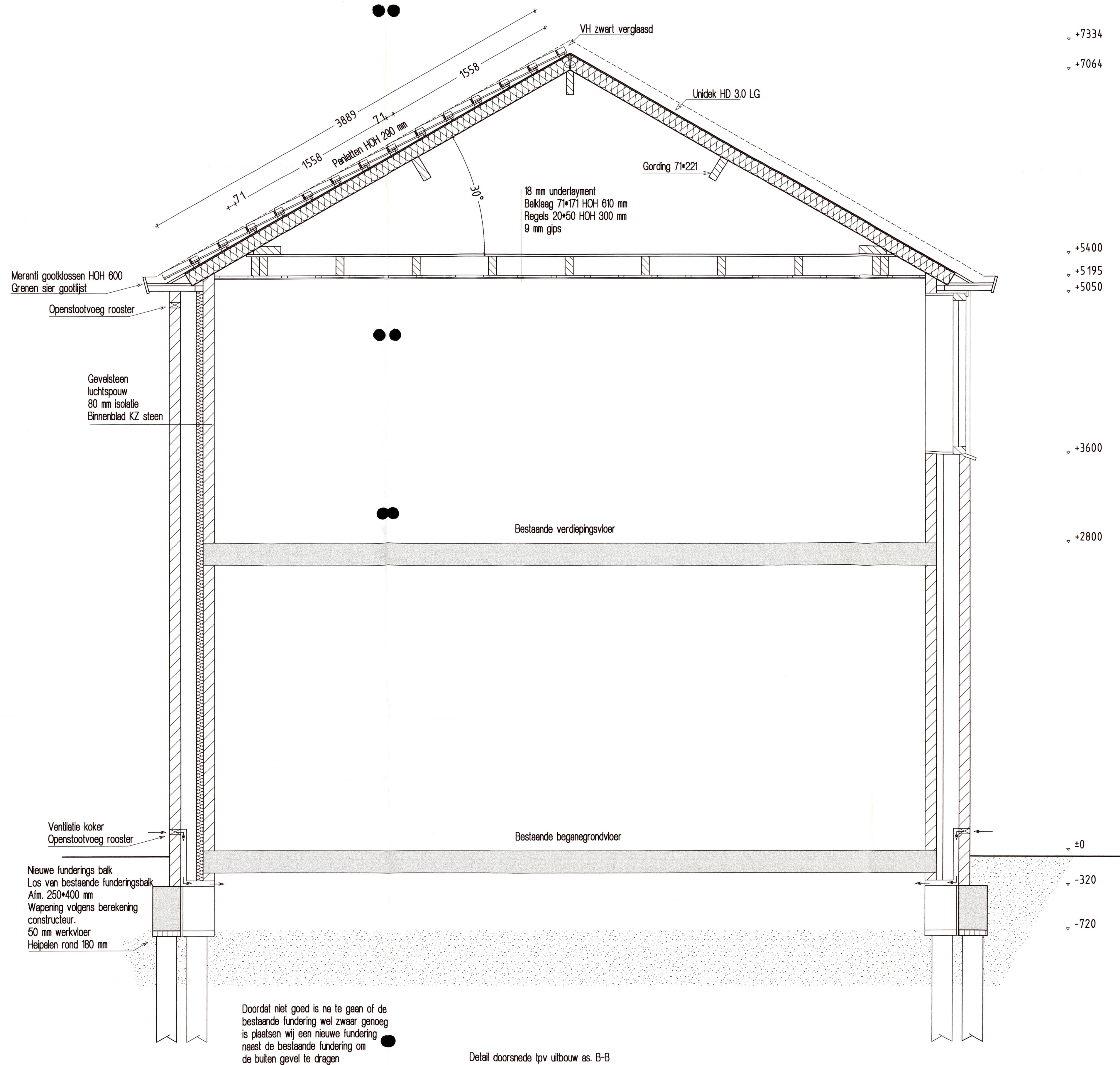
Detail doorsnede tpv uitbouw as. B-B
