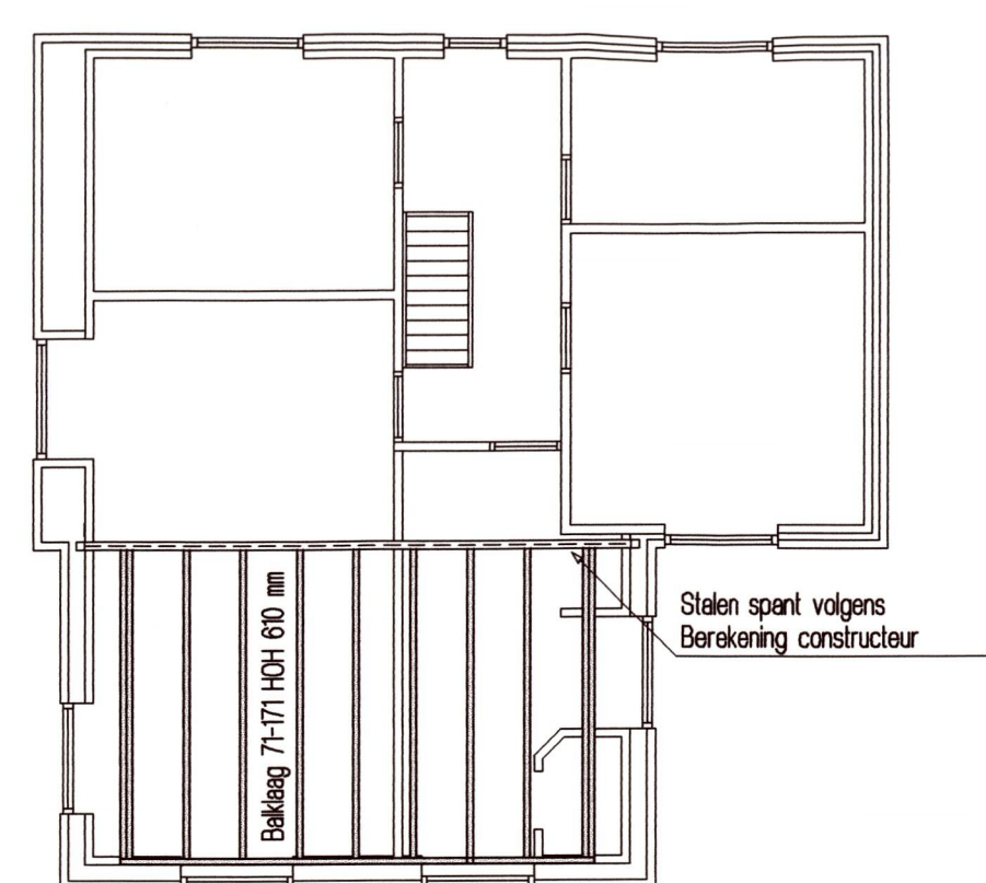
zolder beklaag
