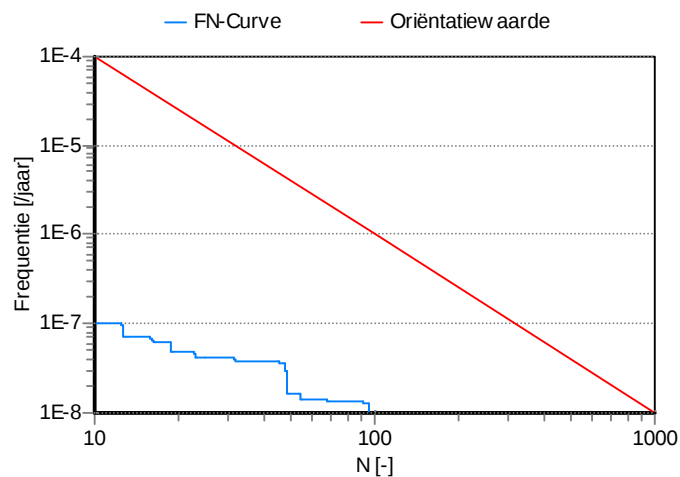
Figuur 5 FN-curve worst-casesegment N-501-25-KR-024 t/m 027, bestaande situatie. Overschrijdingsfactor 0.01.
