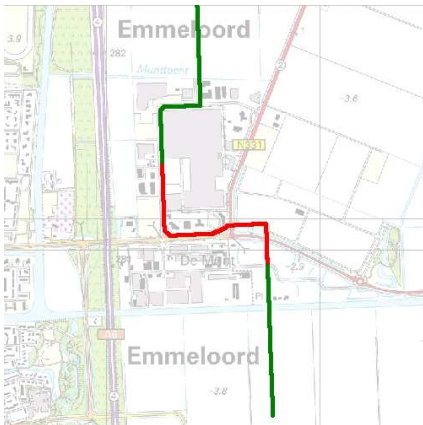
Figuur 6 Worst-casesegment van de N-501-25-KR-024 t/m 027, weergegeven in rood. Dit segment levert het hoogste groepsrisico op in de nieuwe situatie.
