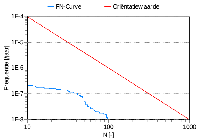
Figuur 3 FN-curve worst-casesegment N-501-25-KR-024 t/m 027, nieuwe situatie. Overschrijdingsfactor 0.02.
