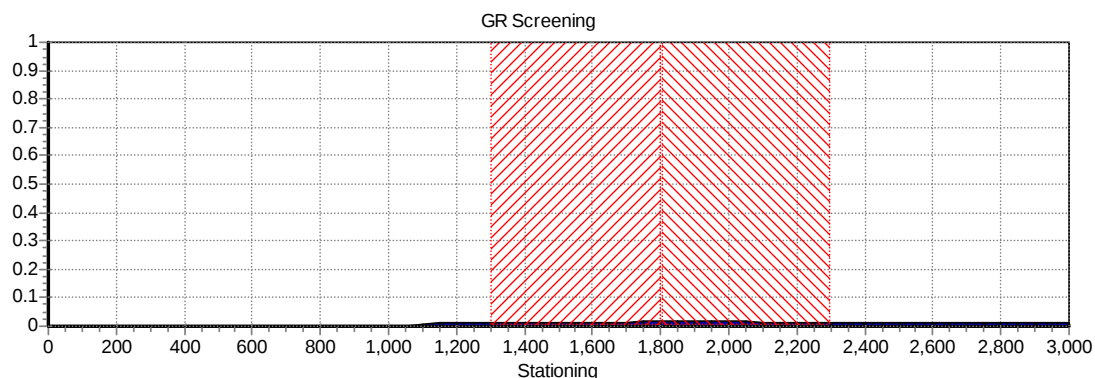
Figuur 2 Overschrijdingsfactor uitgezet tegen stationing van de N-501-25-KR-024 t/m 027, nieuwe situatie. Het rood gearceerde deel geeft de kilometer aan waarover de FN-curve is berekend.
