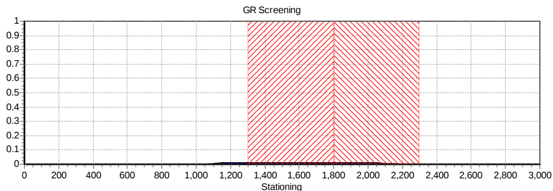
Figuur 4 Overschrijdingsfactor uitgezet tegen stationing van de N-501-25-KR-024 t/m 027, bestaande situatie. Het rood gearceerde deel geeft de kilometer aan waarover de FN-curve is berekend.
