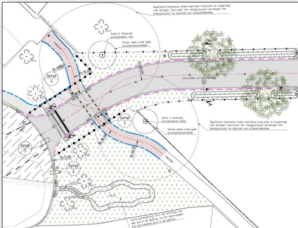
Foto 3: bovenaanzicht ontwerpplan Ambachtstraat De Lutte. Bron; Gemeente Losser, bewerking Expedio Arbori
