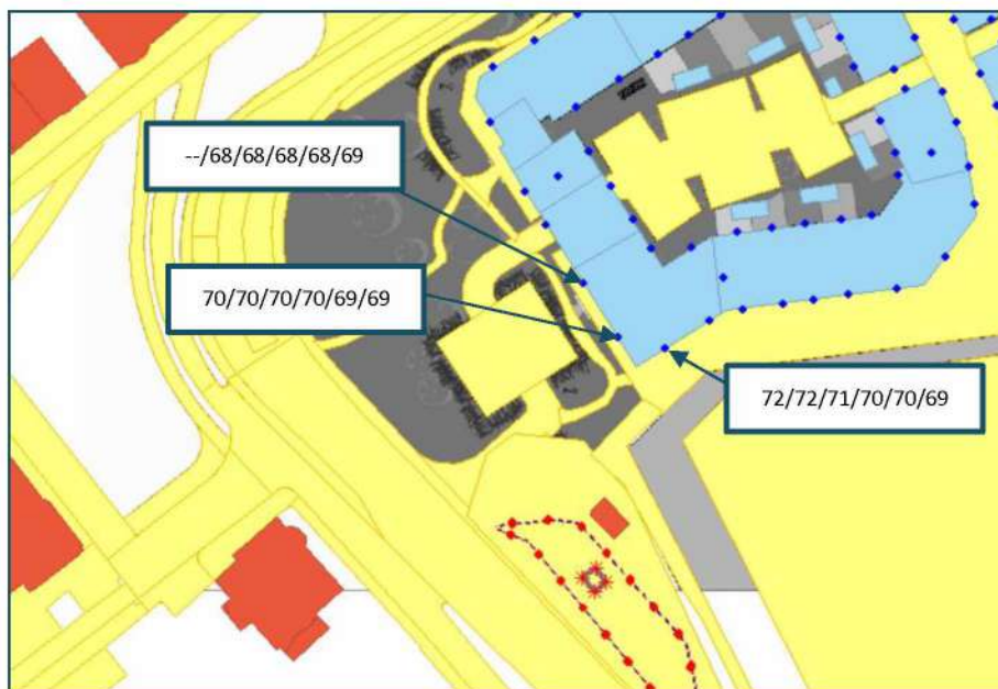
Figuur 6 Maximale geluidniveaus op de maatgevende gevels op begane grond en bovenliggende verdiepingen in de nachtperiode
