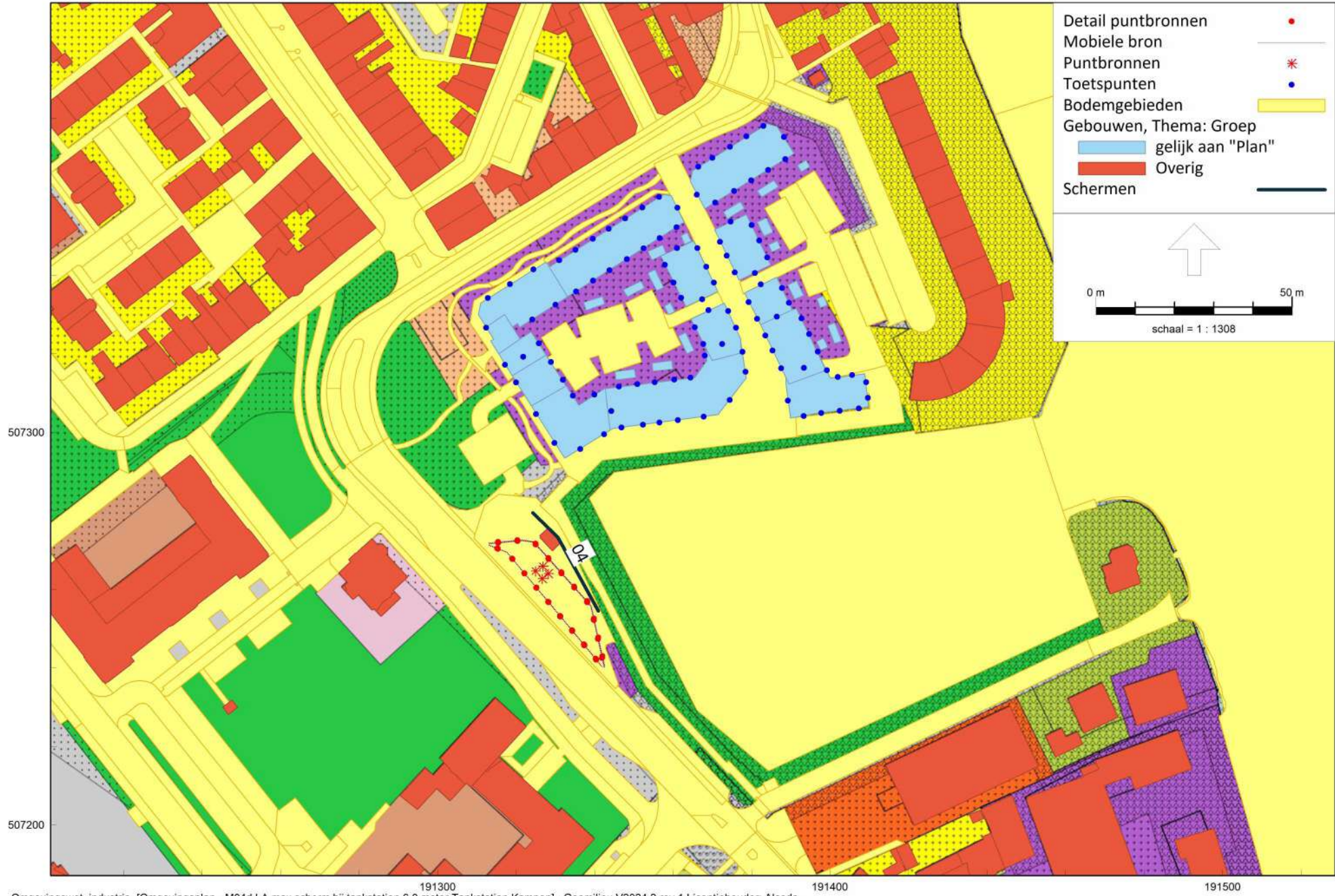
Ligging scherm bij tankstation
