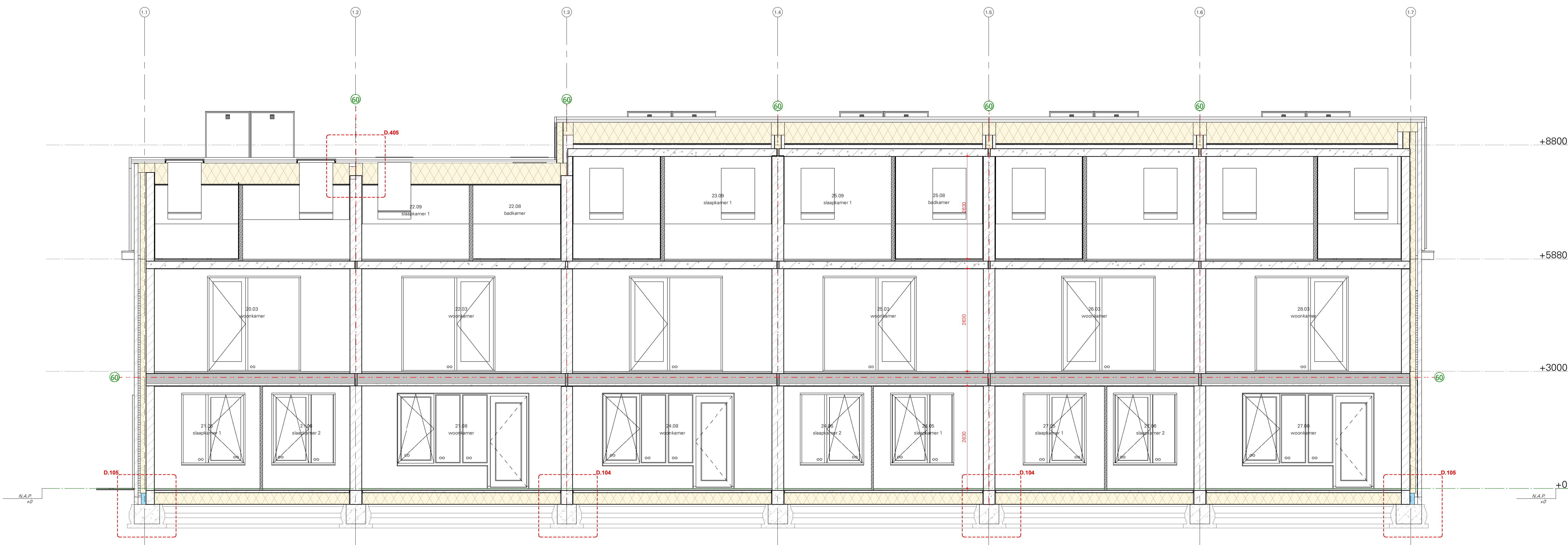
Doorsnede A - Blok 1
