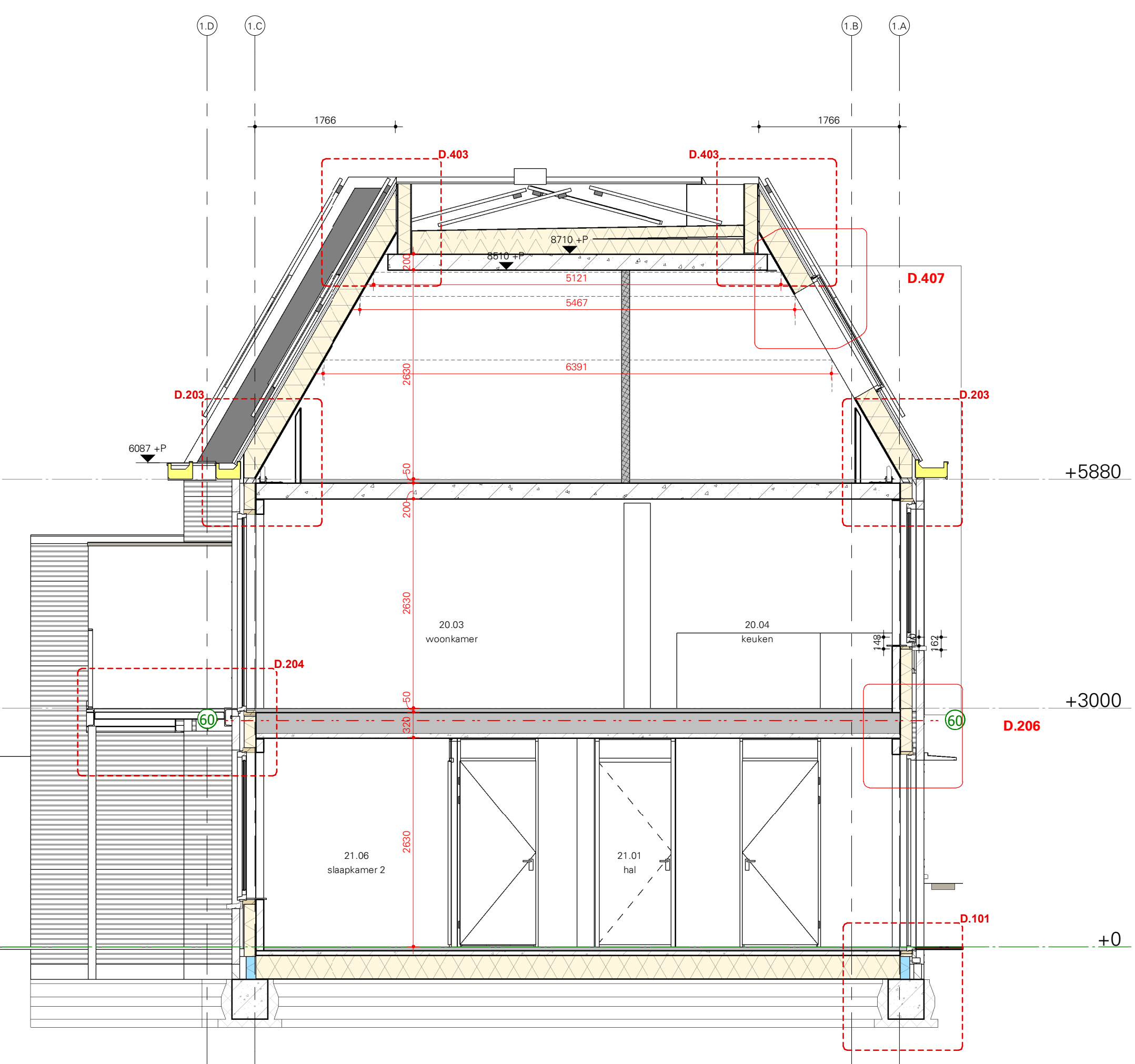
Doorsnede C - Blok 1
