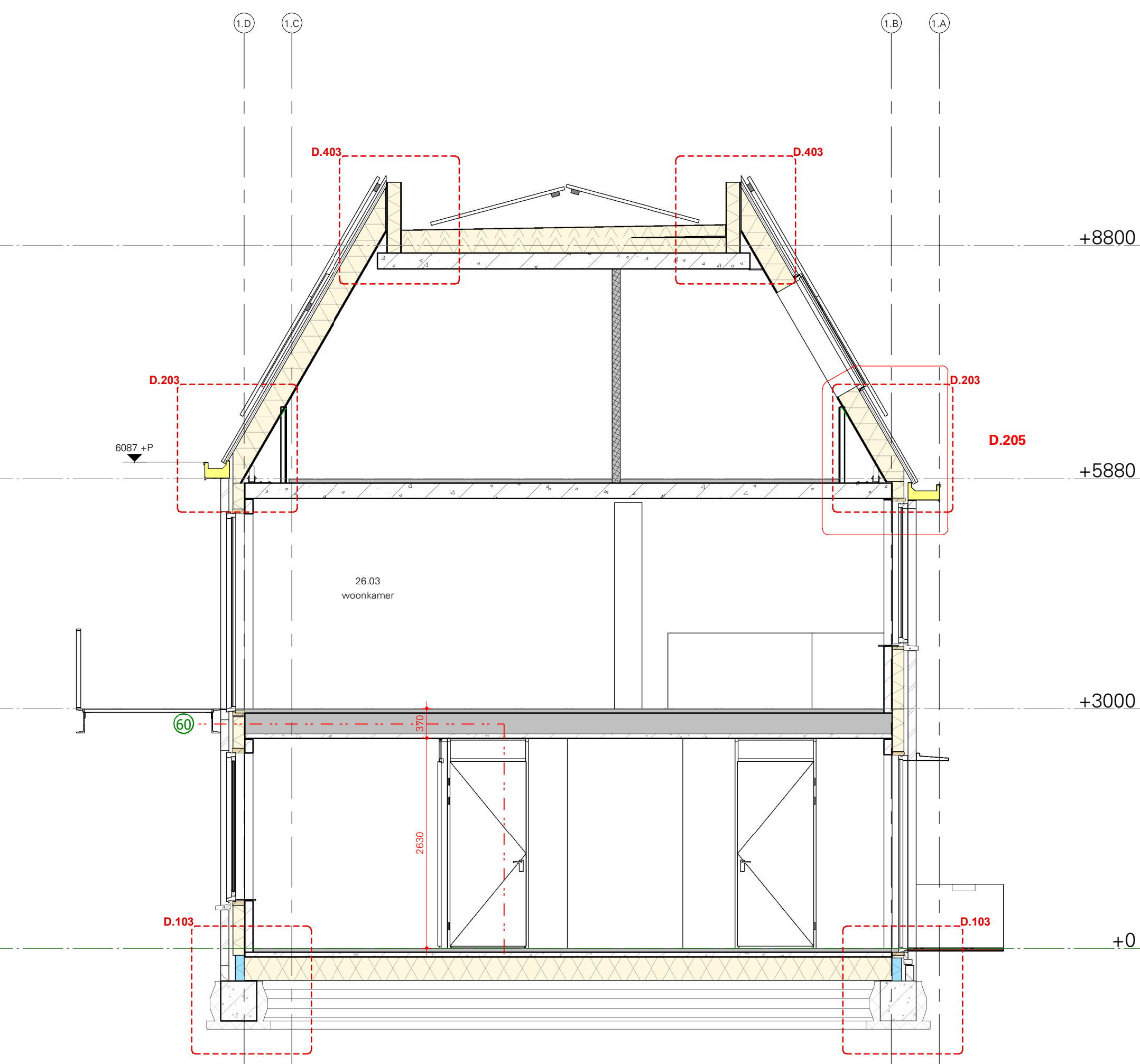
Doorsnede D - Blok 1
