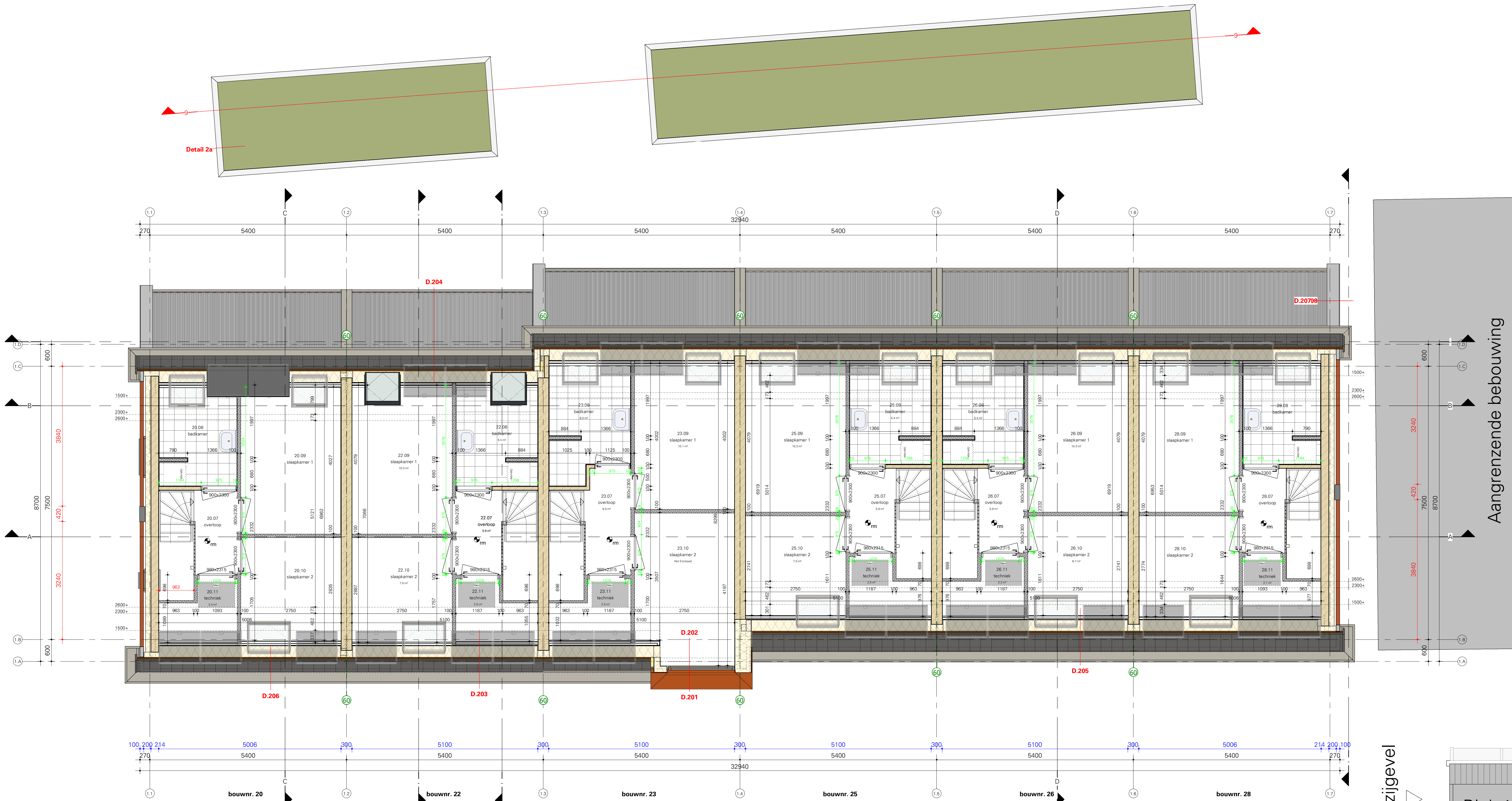
Plattegrond tweede verdieping - Blok 1
