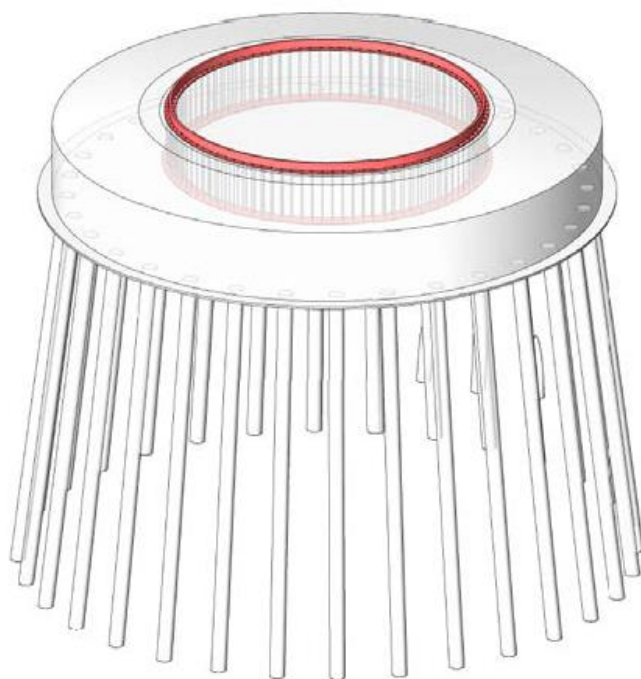
Figuur 3.5 Schematische weergave paalfundering windturbine
