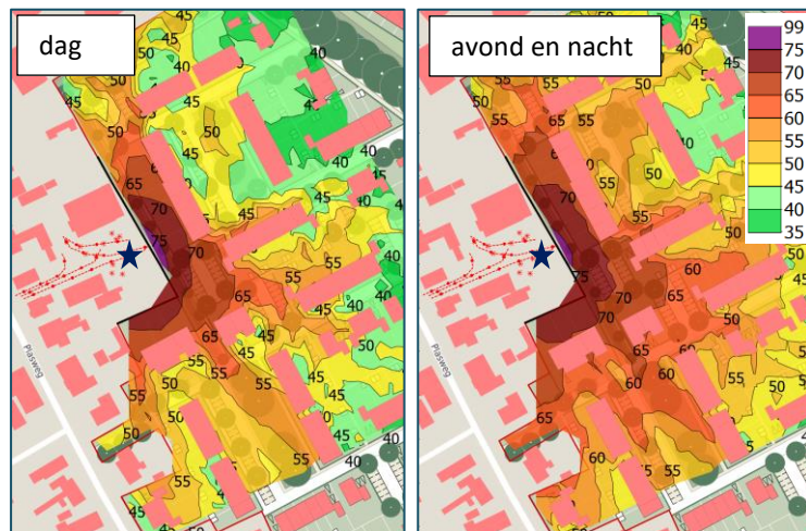
Figuur 8 Maximale geluidsniveaus ( L_{Amax} ) – bronpositie 2
