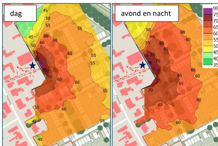
Figuur 3 Maximale geluidsniveaus ( L_{Amix} ) in vrije-veld situatie – bronpositie 1
