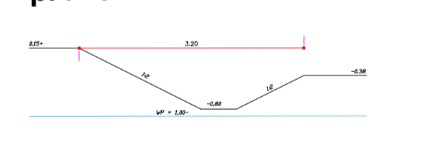
profiel 2
