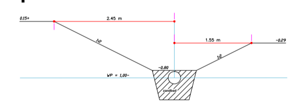
profiel 2
