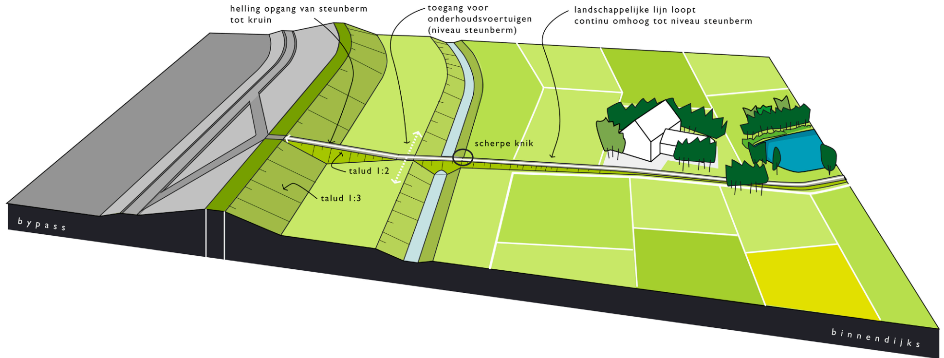
Principes op- afrit binnendijks
