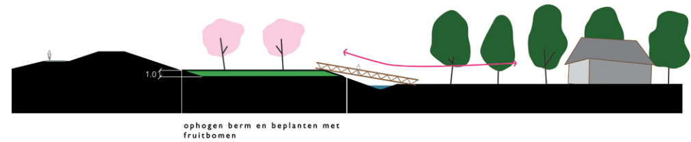
MAAR ZO gebruik binnenberm: 1 m. ophogen en beplanten met fruitbomen, ontwikkel relatie met achterliggende bebouwing
