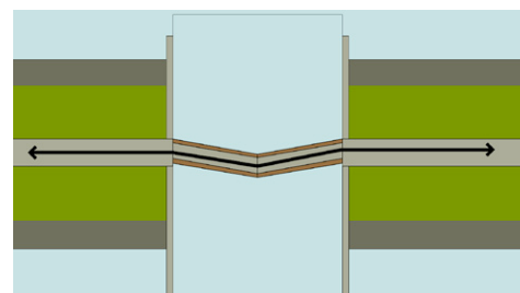
Sluisdeuren als fietsverbinding, liggen exact in lijn met de kruin van de dam
