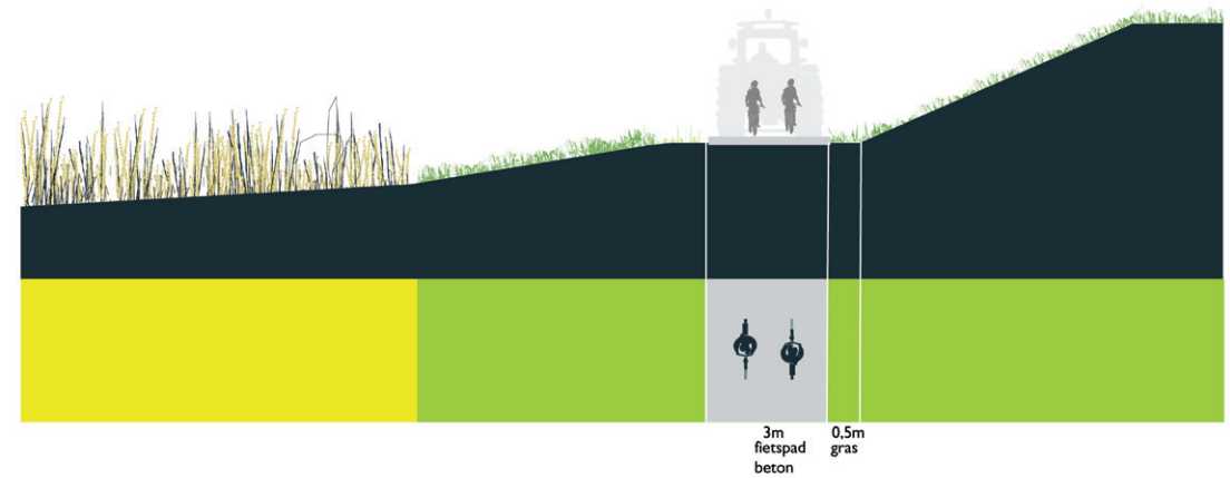
B. Profiel voet-fietspad rond kanteldijk thv rietmilieus
