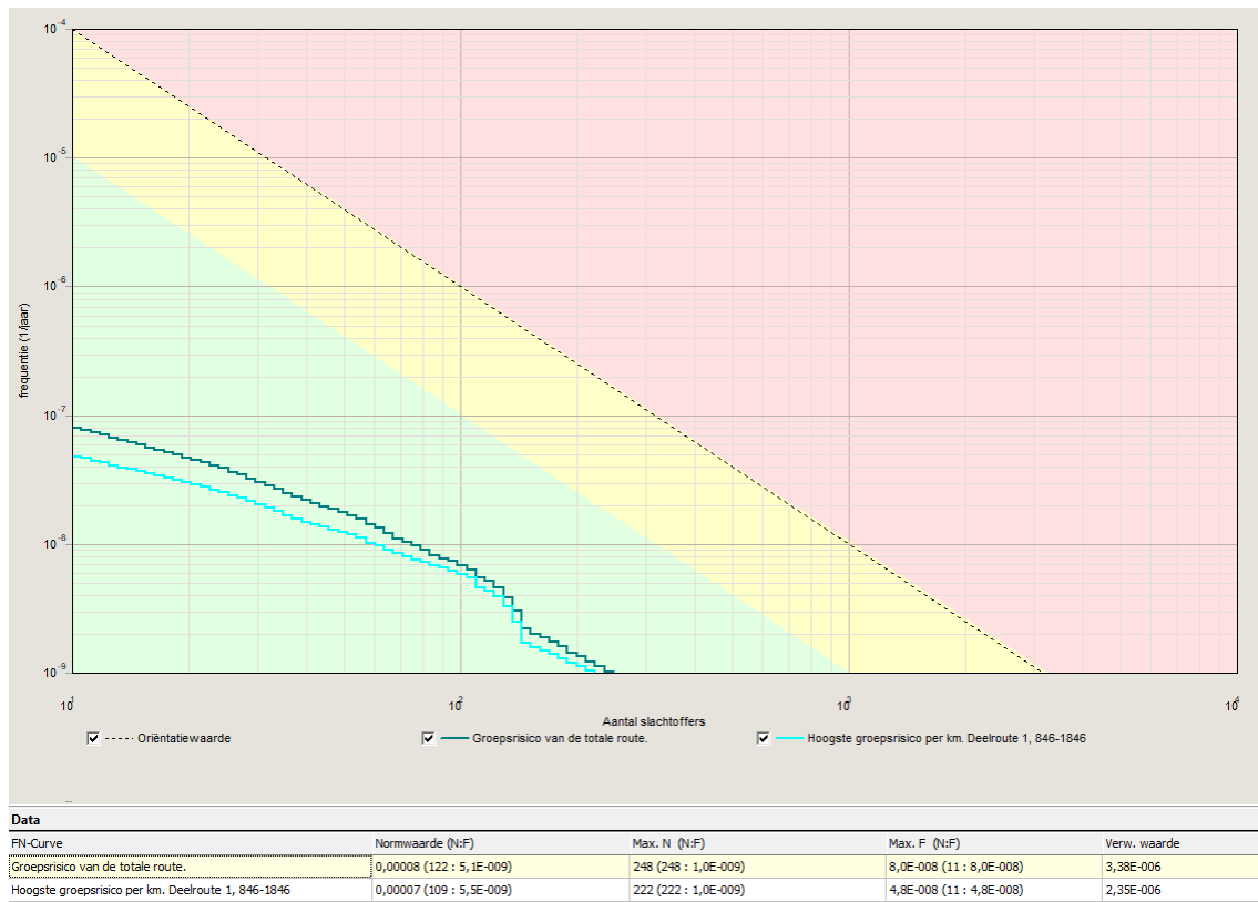
Afbeelding 4 fN-curve berekend groepsrisico, toekomstige situatie
