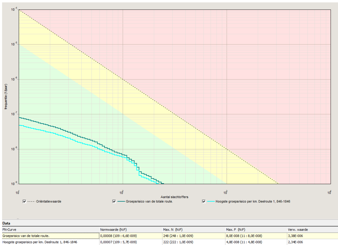
Afbeelding 2 fN-curve berekend groepsrisico - huidige situatie
