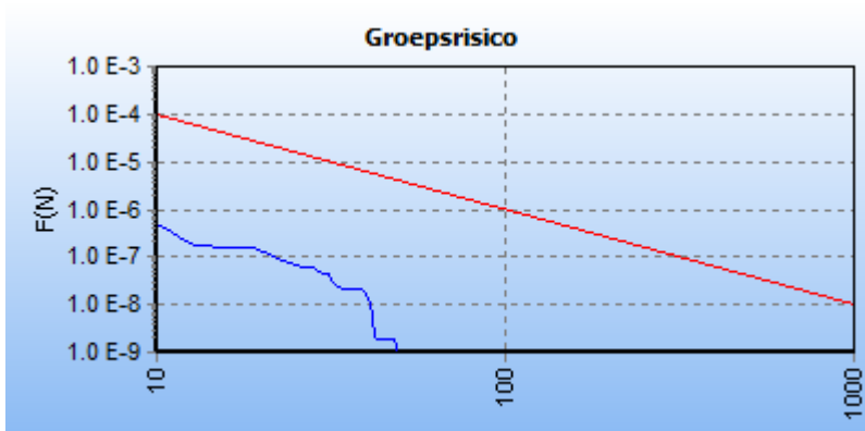
5.2 Figuur 5.2 FN curve voor 618_leiding-N-528-66-deel-1 van N.V. Nederlandse Gasunie voor de kilometer tussen stationing 1000.00 en stationing 2000.00
