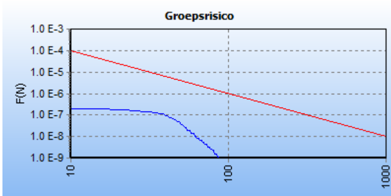
5.1 Figuur 5.1 FN curve voor 618_leiding-A-508-04-deel-1 van N.V. Nederlandse Gasunie voor de kilometer tussen stationing 1120.00 en stationing 2120.00
