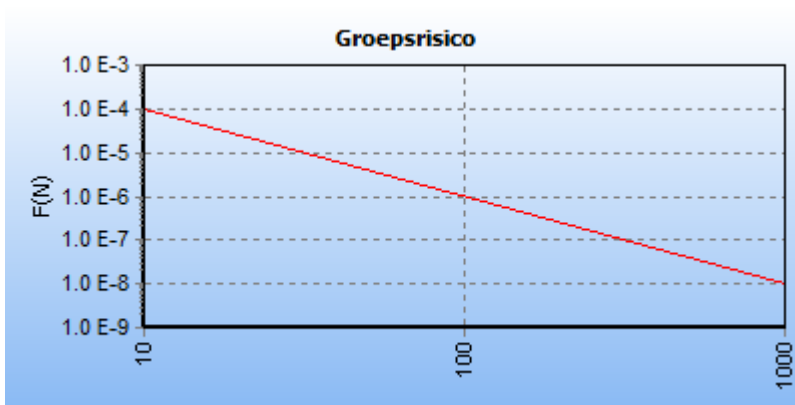
5.1 Figuur 5.1 FN curve voor 598_leiding-A-670-deel-1 van N.V. Nederlandse Gasunie voor de kilometer tussen stationing 1110.00 en stationing 2110.00
