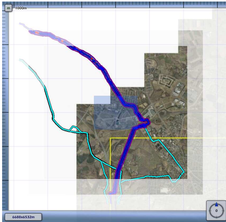
3.2 Figuur 3.2 Plaatsgebonden risico voor 598_leiding-N-528-70-deel-1 van N.V. Nederlandse Gasunie
