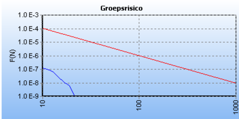
5.1 Figuur 5.1 FN curve voor A-508 van N.V. Nederlandse Gasunie voor de kilometer tussen stationing 42880.00 en stationing 43880.00
