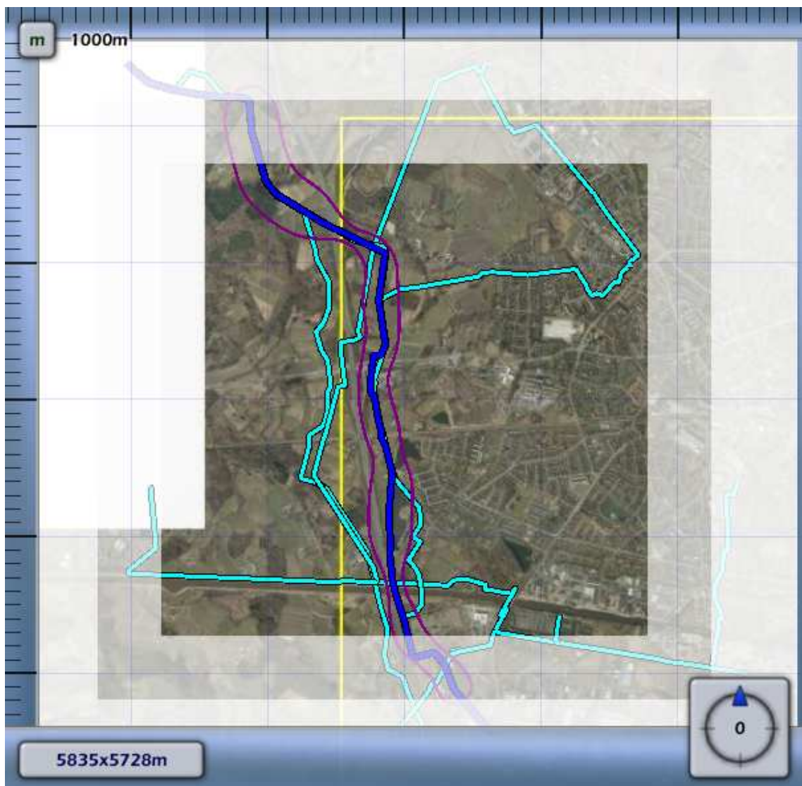
3.2 Figuur 3.2 Plaatsgebonden risico voor A-646 van N.V. Nederlandse Gasunie
