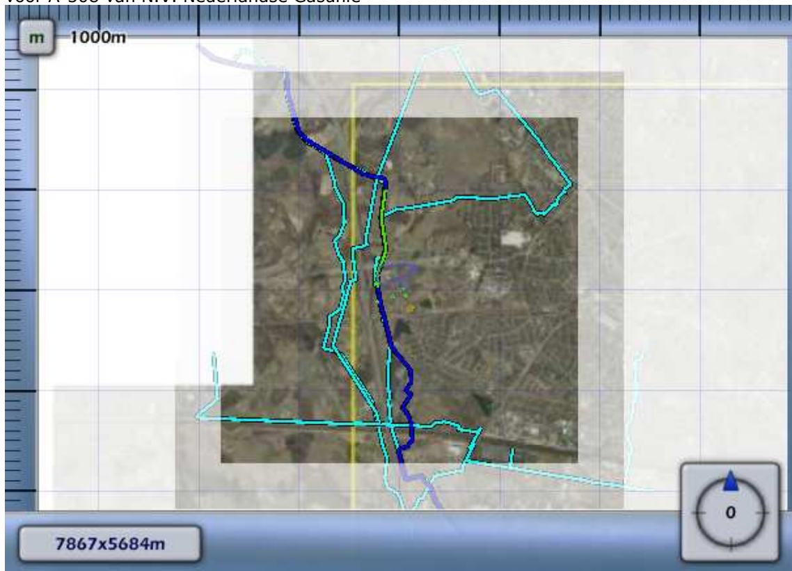
Figuur 4.2 Kilometer leiding behorende bij de maximale overschrijding van de FN-curve voor A-508 van N.V. Nederlandse Gasunie
