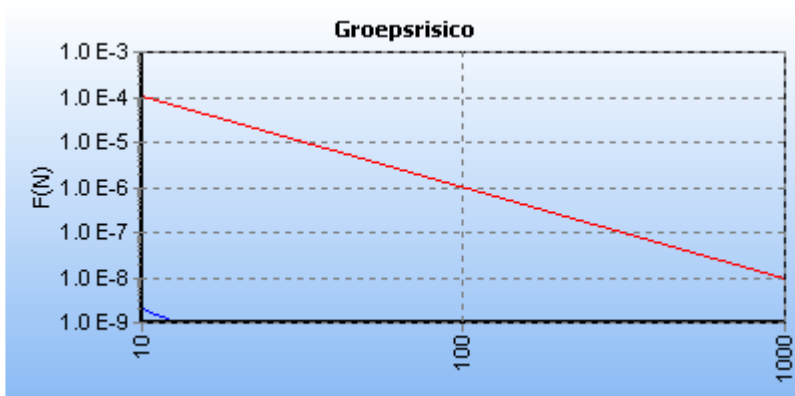
5.2 Figuur 5.2 FN curve voor A-646 van N.V. Nederlandse Gasunie voor de kilometer tussen stationing 7320.00 en stationing 8320.00
