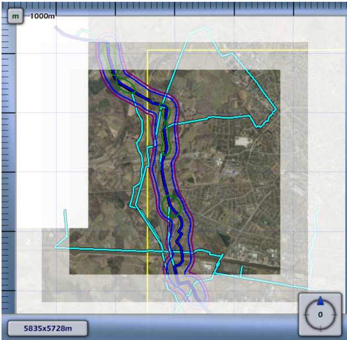
3.1 Figuur 3.1 Plaatsgebonden risico voor A-508 van N.V. Nederlandse Gasunie
