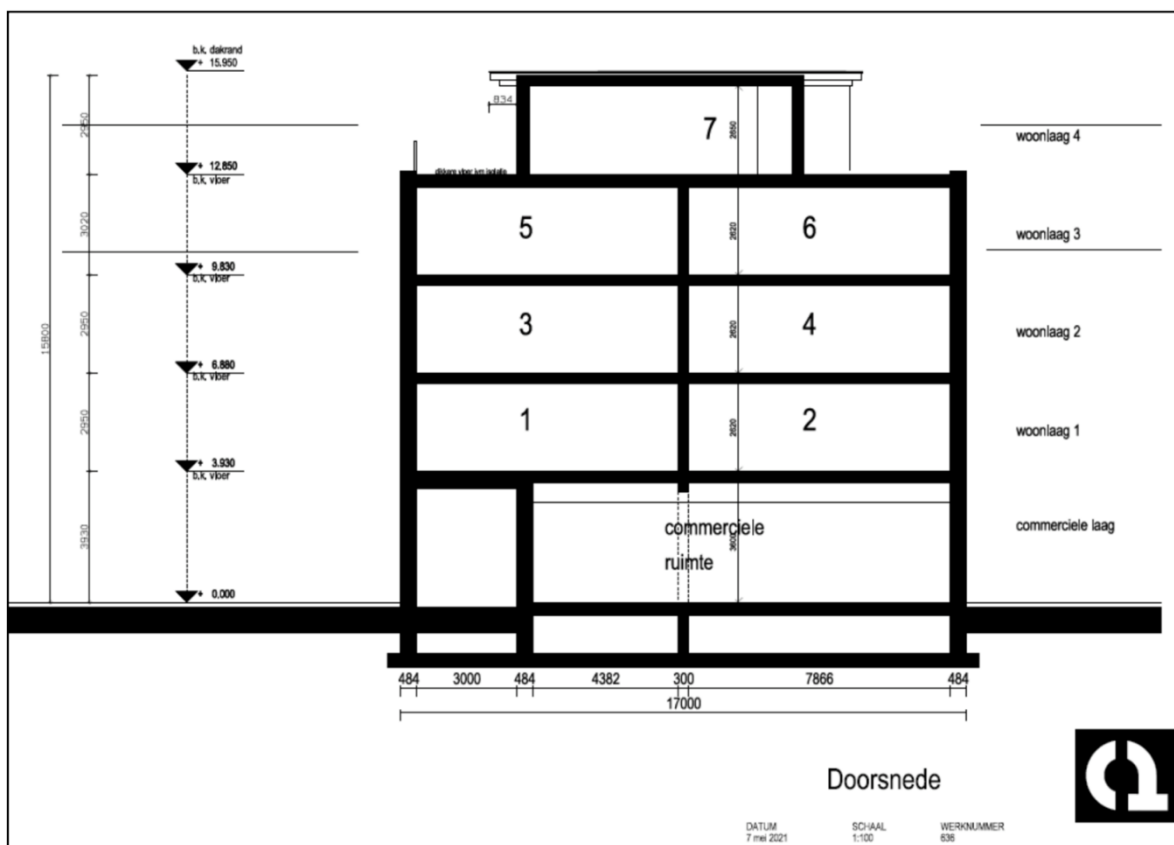
Afbeelding 3.2 Doorsnede gebouw nieuwe situatie (Bron: 01 Architecten)
