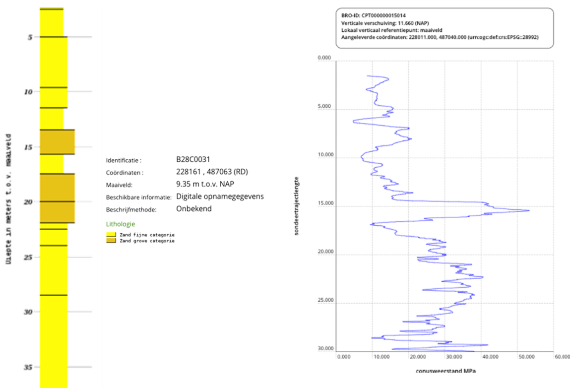
Figuur 2 Boring (links) en sondering (rechts)
