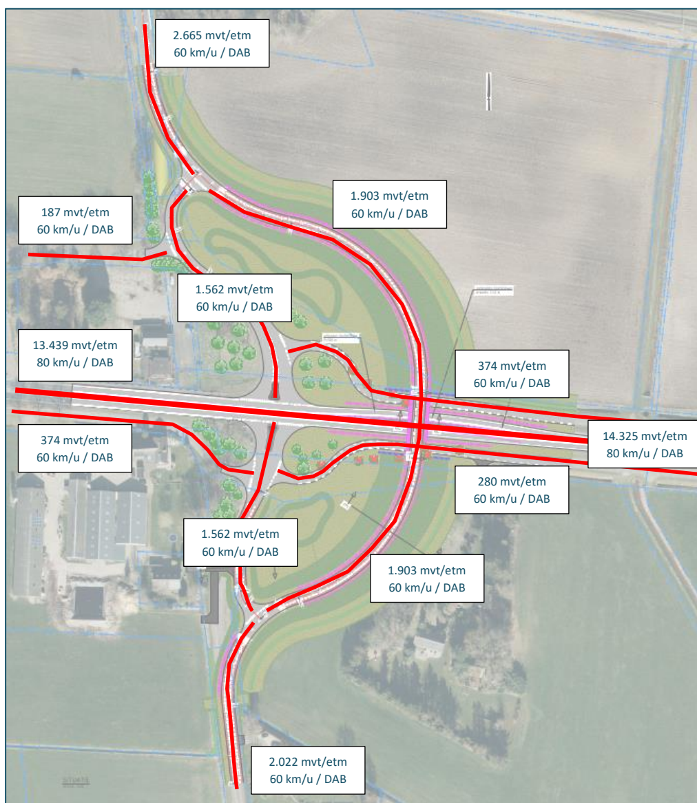
Figuur 5 Verkeers- en verhardingsgegevens 2036
