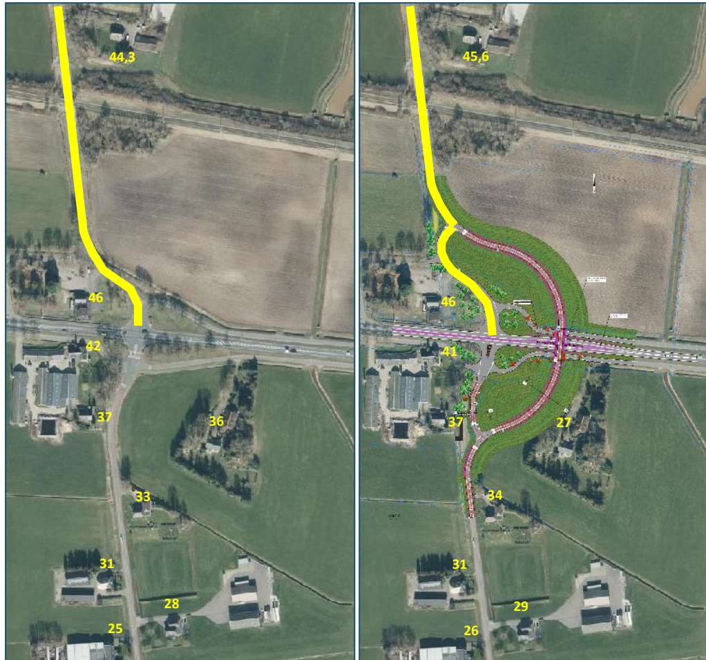
Figuur 13 Geluidbelasting Stationsweg noord
