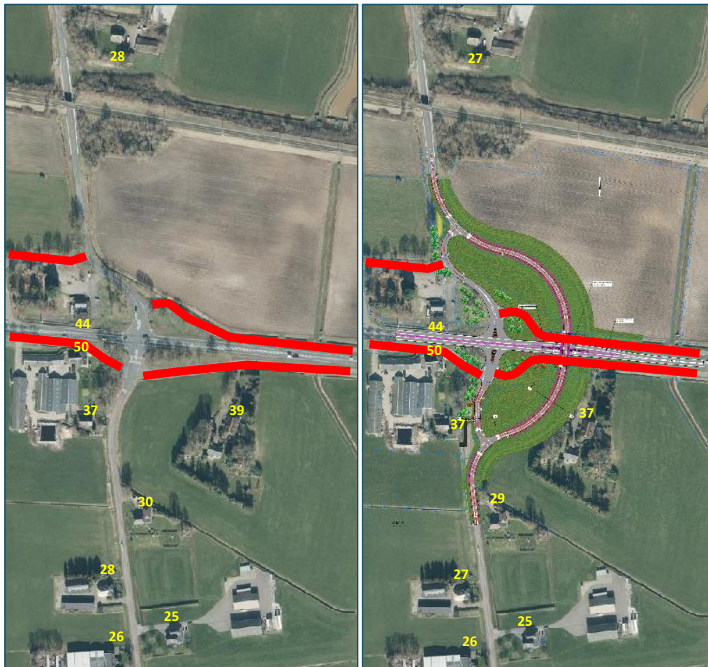
Figuur 15 Geluidbelasting Almeloseweg gezamenlijke parallelwegen
