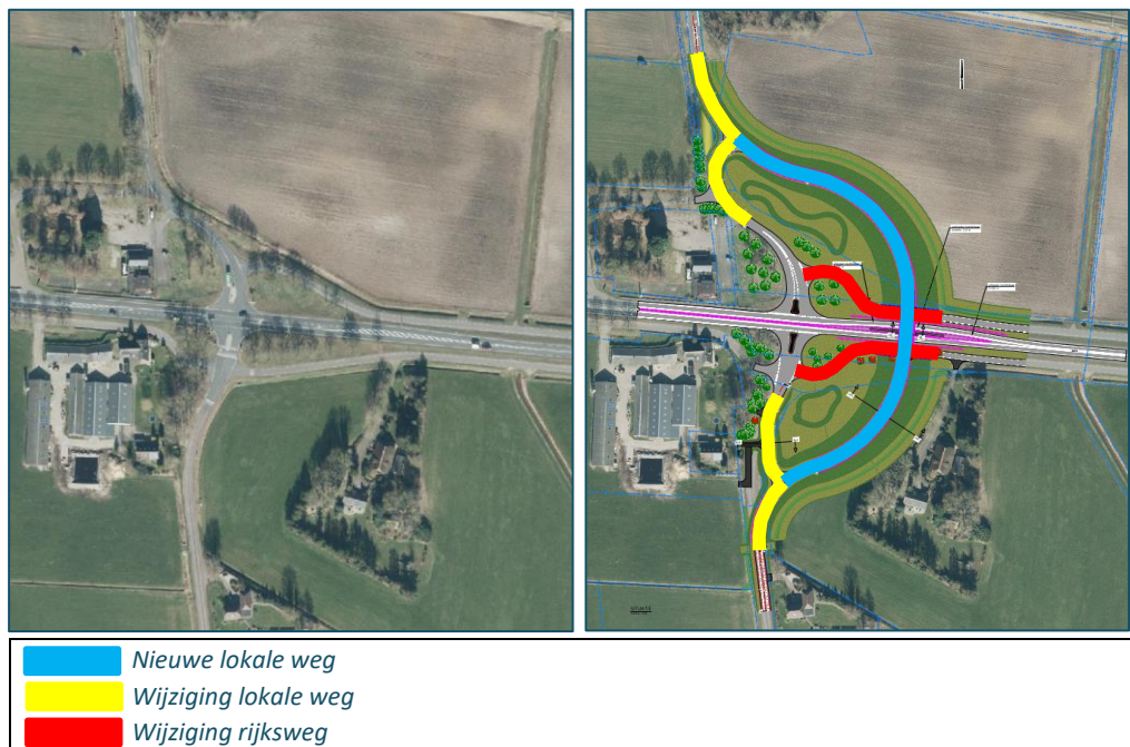
Figuur 3 Gewijzigde en nieuwe wegvakken
