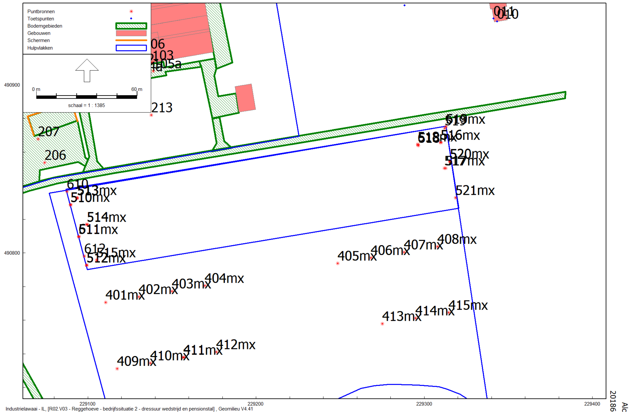
Figuur 3 Bedrijfssituatie 2 ligging van geluidbronnen noordzijde
