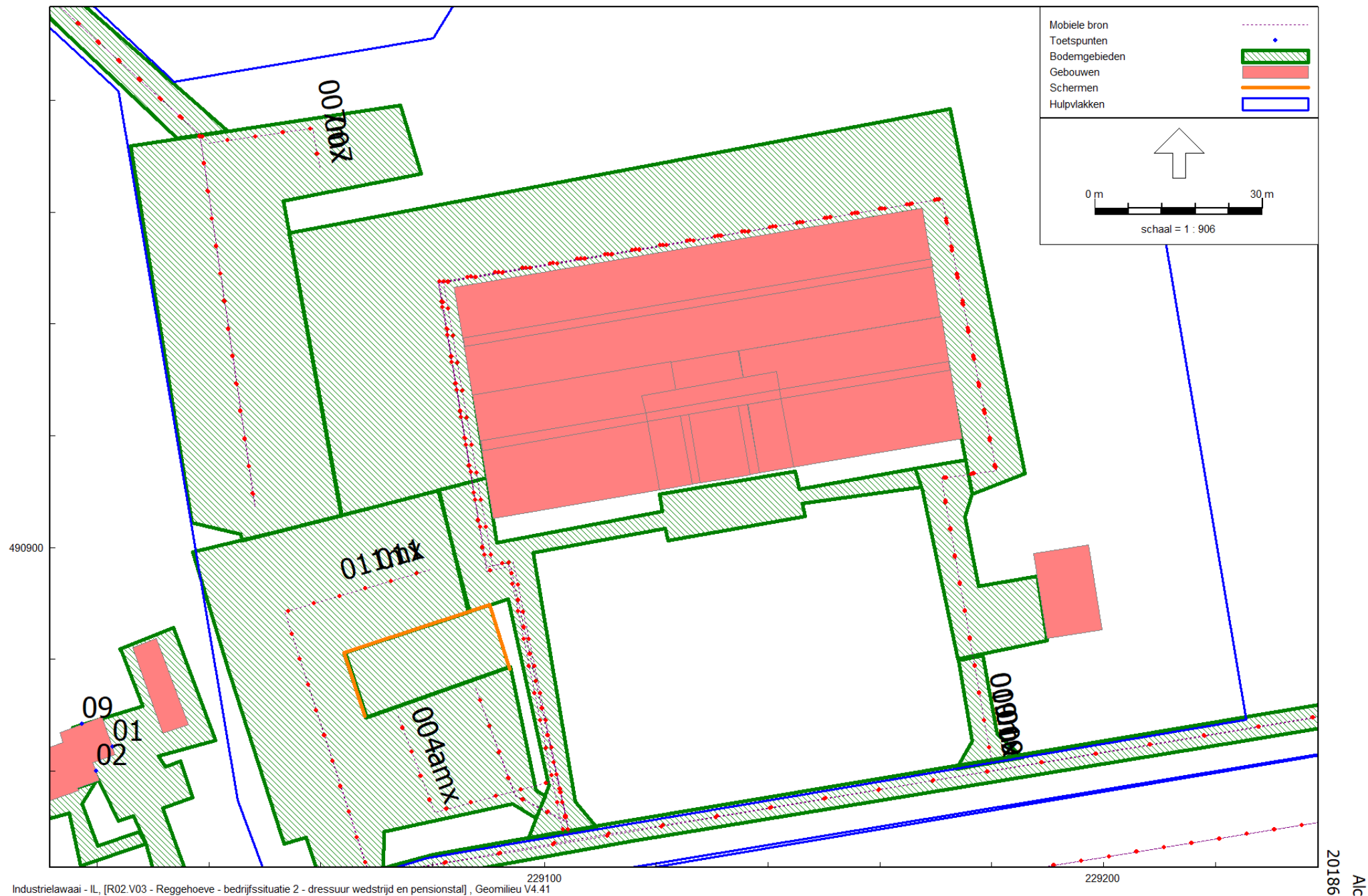
Figuur 4 Bedrijfssituatie 2 ligging van mobiele geluidbronnen noordzijde
