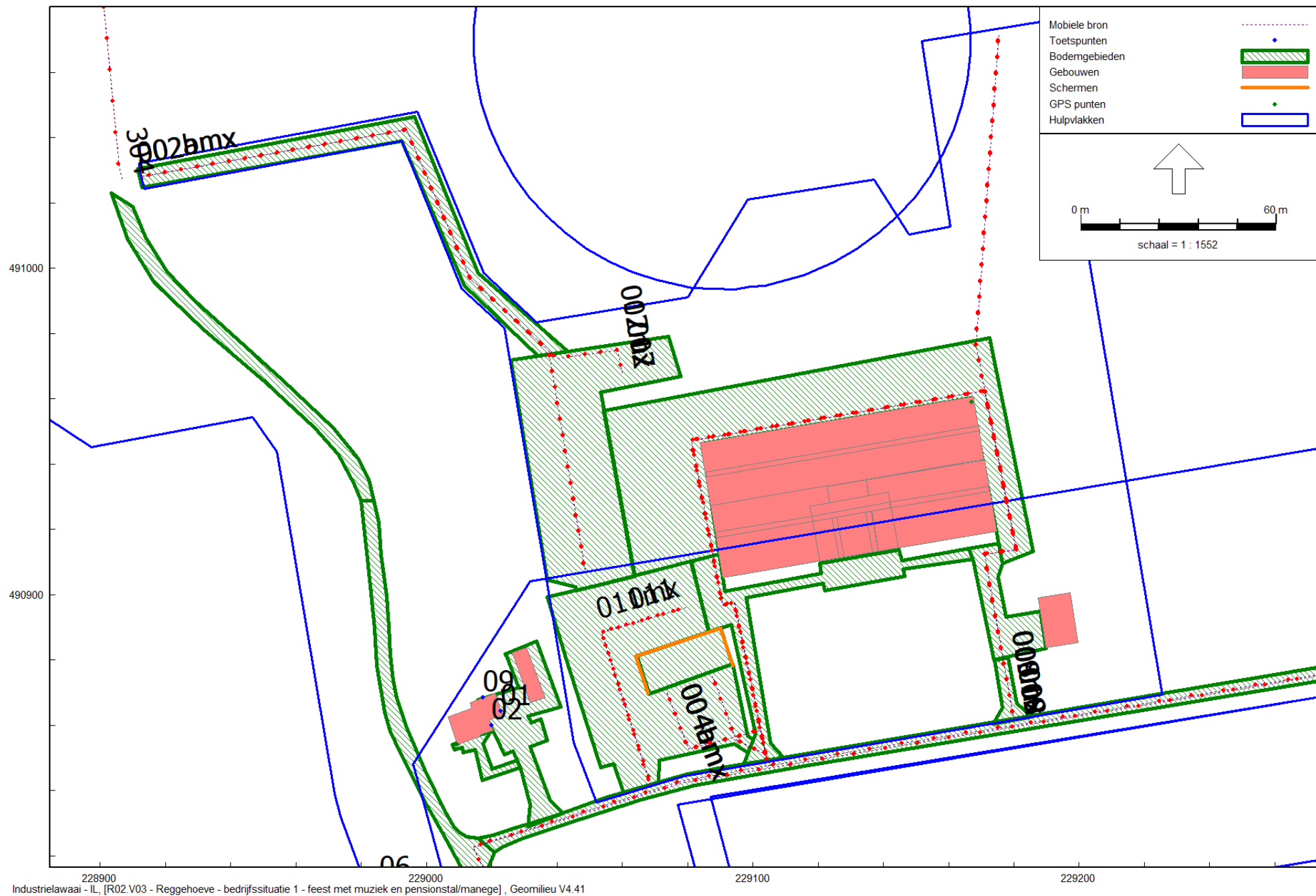
Figuur 2b Bedrijfssituatie 1 Ligging van mobiele geluidbronnen
