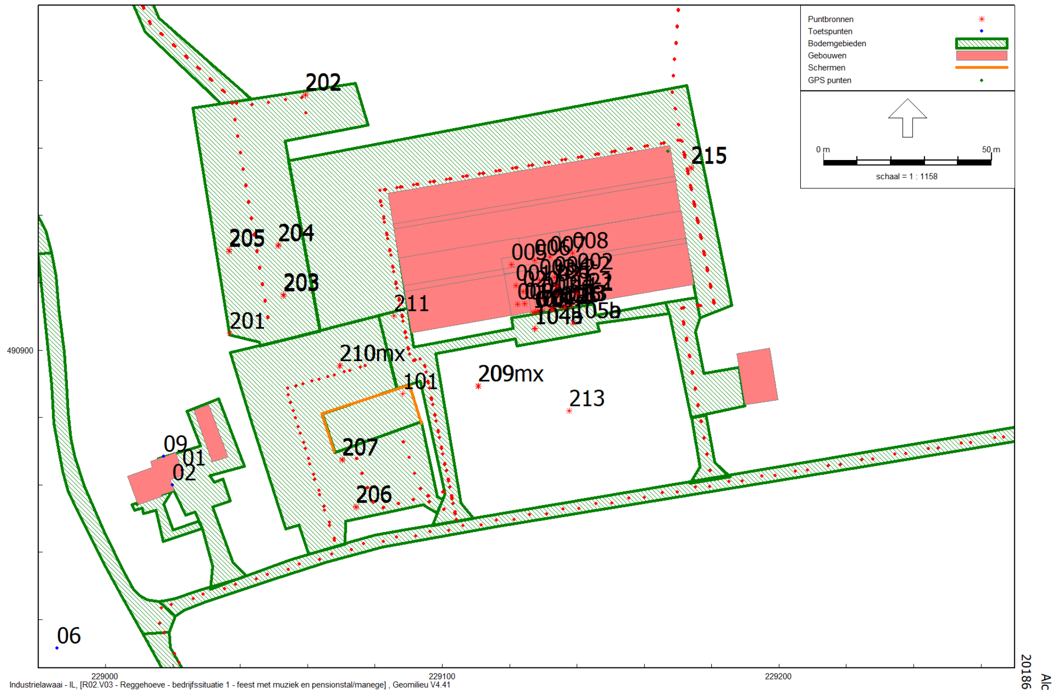
Figuur 2 Bedrijfssituatie 1 Ligging van stationaire geluidbronnen
