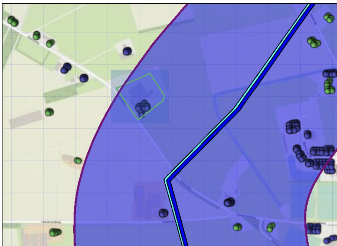
Figuur 3.1 Plaatsgebonden risico voor 8961_leiding-A-523-deel-1 van N.V. Nederlandse Gasunie
