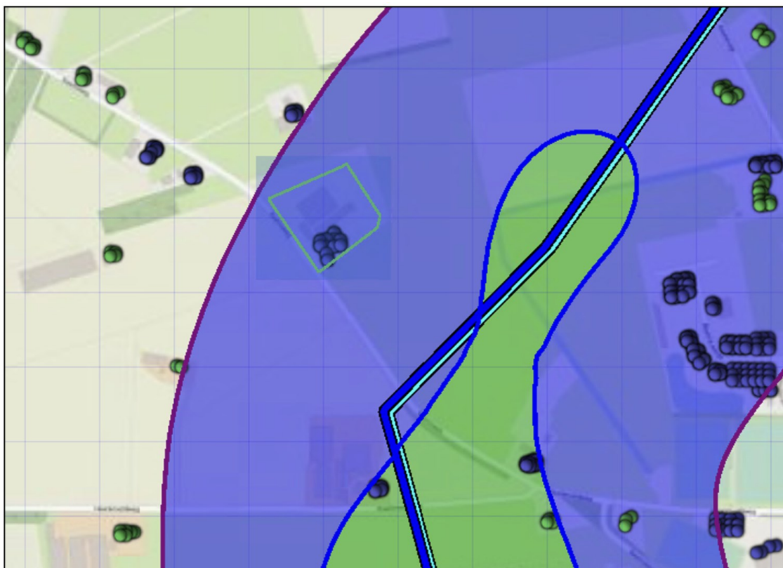
Figuur 3.2 Plaatsgebonden risico voor 8961_leiding-A-529-deel-1 van N.V. Nederlandse Gasunie
