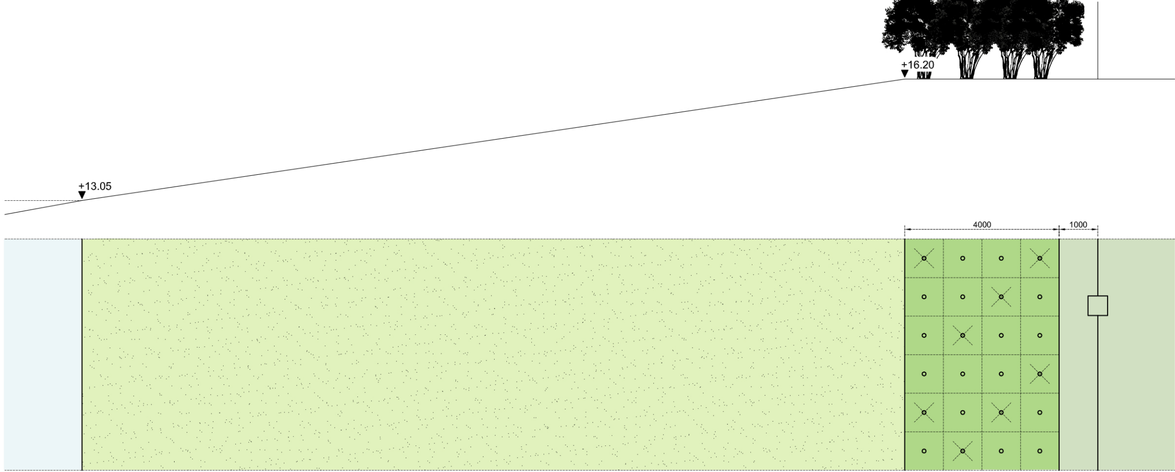
Doorsnede A-A', bosschage 33% uitdunnen na 5 jaar, schaal 1:100
