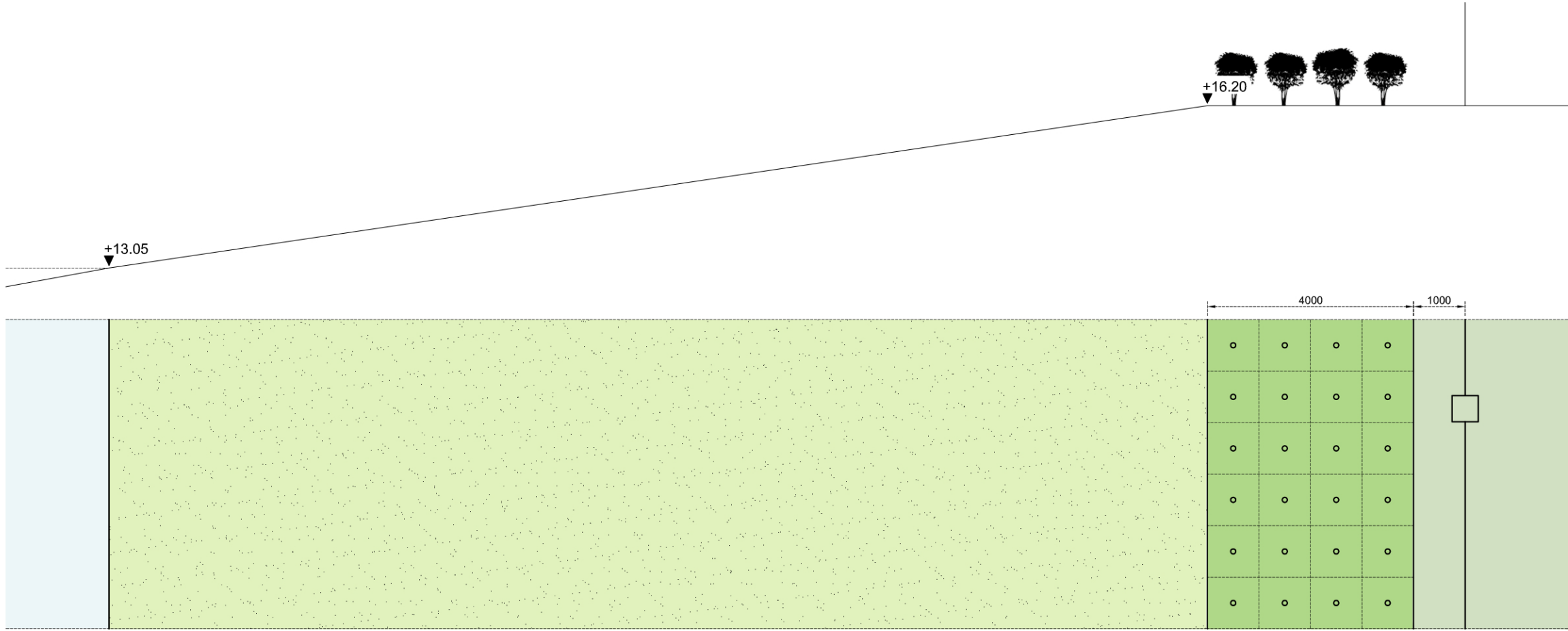
Doorsnede A-A', aanplant bosschage, schaal 1:100
