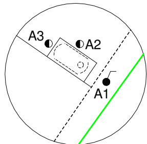
Detailtekening Deellocatie A Schaal 1 : 200
