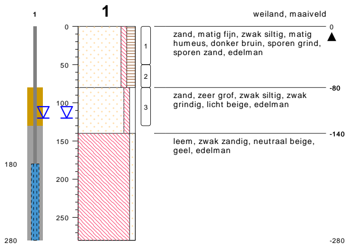
type peilbuis met 1 filter datum 14-04-2020 boormeester Riemer Veltmaat
