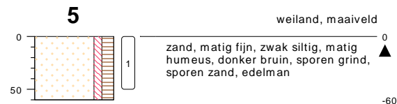
type grondboring datum 14-04-2020 boormeester Riemer Veltmaat
