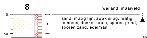
type grondboring datum 14-04-2020 boormeester Riemer Veltmaat
