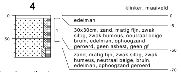
type inspectiegat datum 10-10-2018 boormeester Riemer Veltmaat
