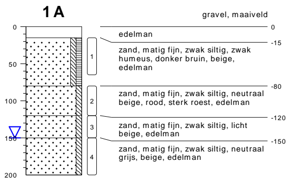
type inspectiegat datum 10-10-2018 boormeester Riemer Veltmaat
