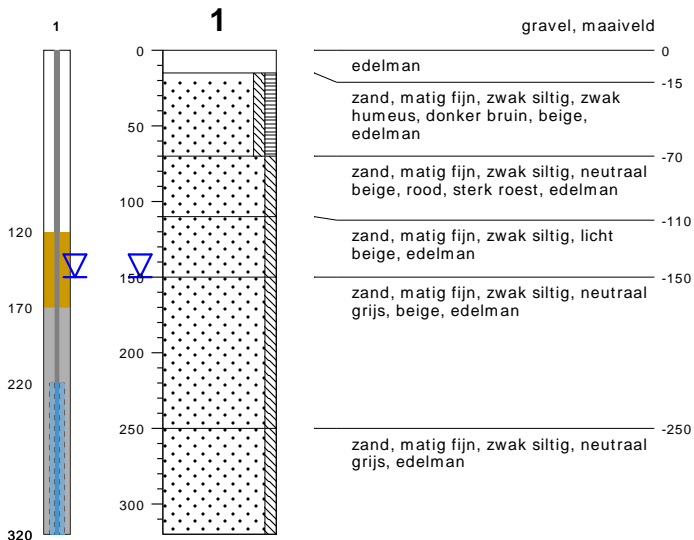
type peilbuis met 1 filter datum 02-10-2018 boormeester Riemer Veltmaat
