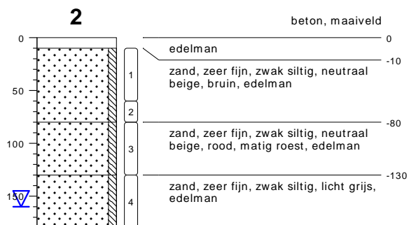
type inspectiegat datum 10-10-2018 boormeester Riemer Veltmaat
