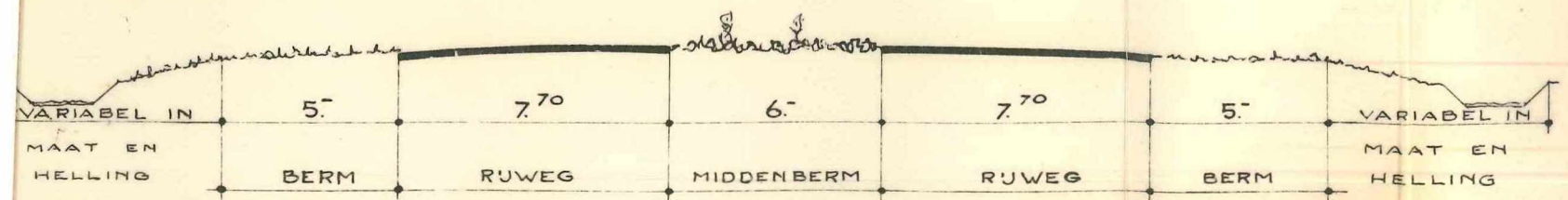
ALGEMEEN DWARSPROFIEL WESTELIJKE INVALSWEG SCHAAL 1:200
