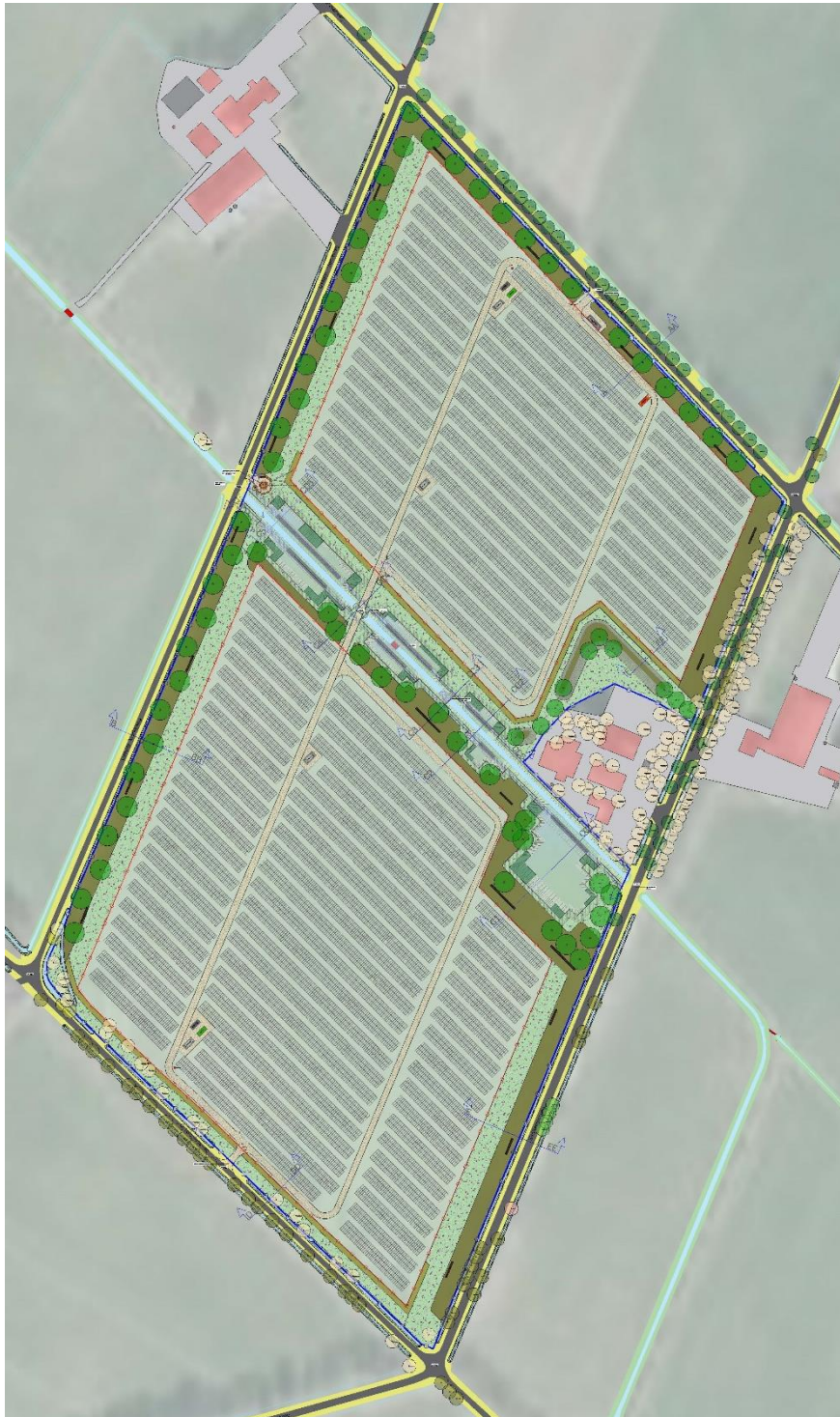
FIGUUR 7: LANDSCAPPELIJK ONTWERP ZONNEPARK BROEKHEURNE, VOOR VOLLEDIGE WEERGAVE ZIE BIJLAGE 1A: LANDSCAPPELIJK ONTWERP. BRON: STUDIO NICO WISSING.
