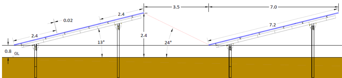
FIGUUR 10: UITSNEDE TECHNISCHE TEKENING VAN DE TE BOUWEN OPSTELLING VAN ZONNEPARK BROEKHEURNE. ZIE BIJLAGE 3A VOOR DE GEHELE WEERGAVE VAN HET TECHNISCH ONTWERP. BRON: TPSOLAR.
