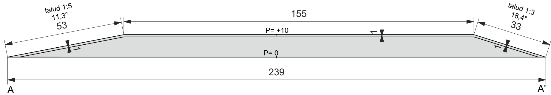
DOORSNEDE A 1:1000
