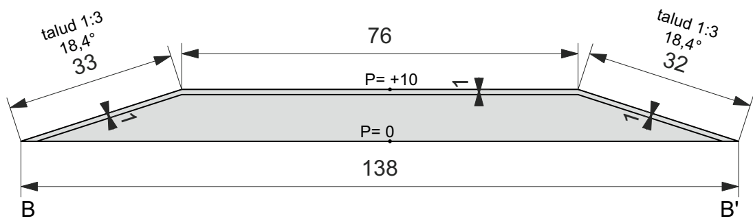
DOORSNEDE B 1:1000
