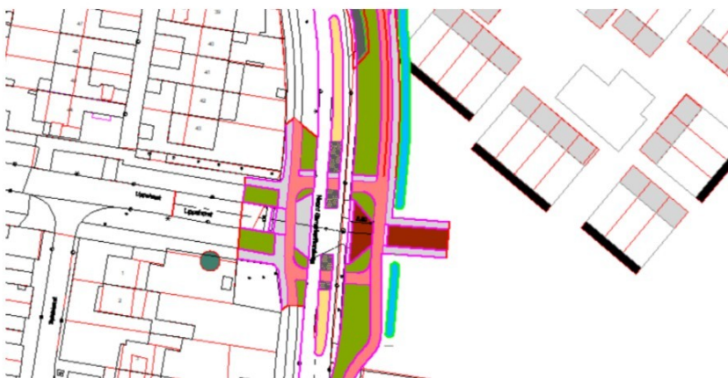
Figuur 3.2: Mogelijk ontwerp voor een westelijke ontsluiting
