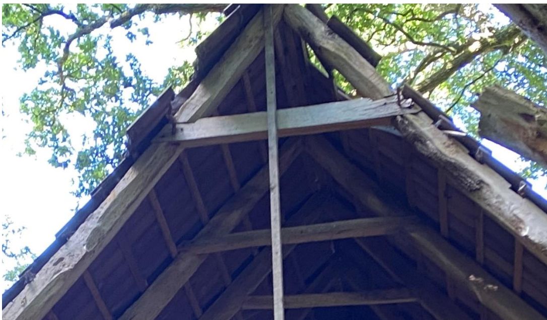
Afb. Kapconstructie met spoorparen en haanhouten, allen voorzien van telmerken.
