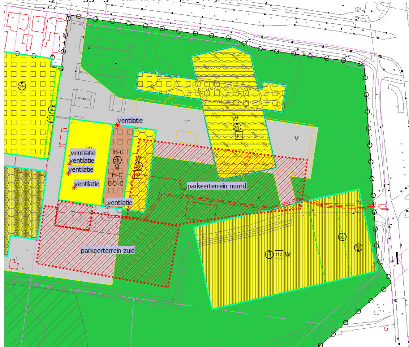
Afbeelding 3.3: ligging installaties en parkeerplaatsen
