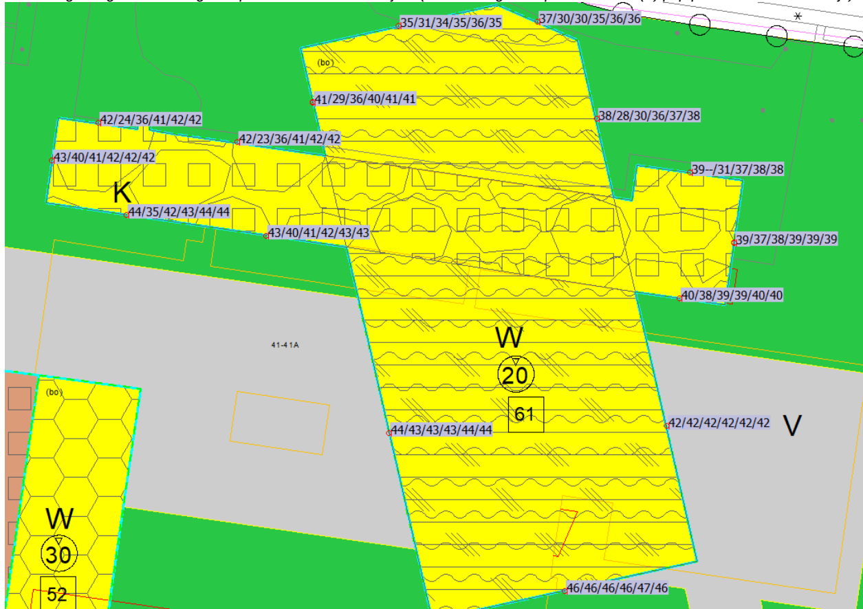
Afbeelding 3.9: geluidbelasting LAeq incidentele situatie 8x jaar (in voormalige drukpershal: 95 dB(A) pop parkeren alleen zuidelijk)
