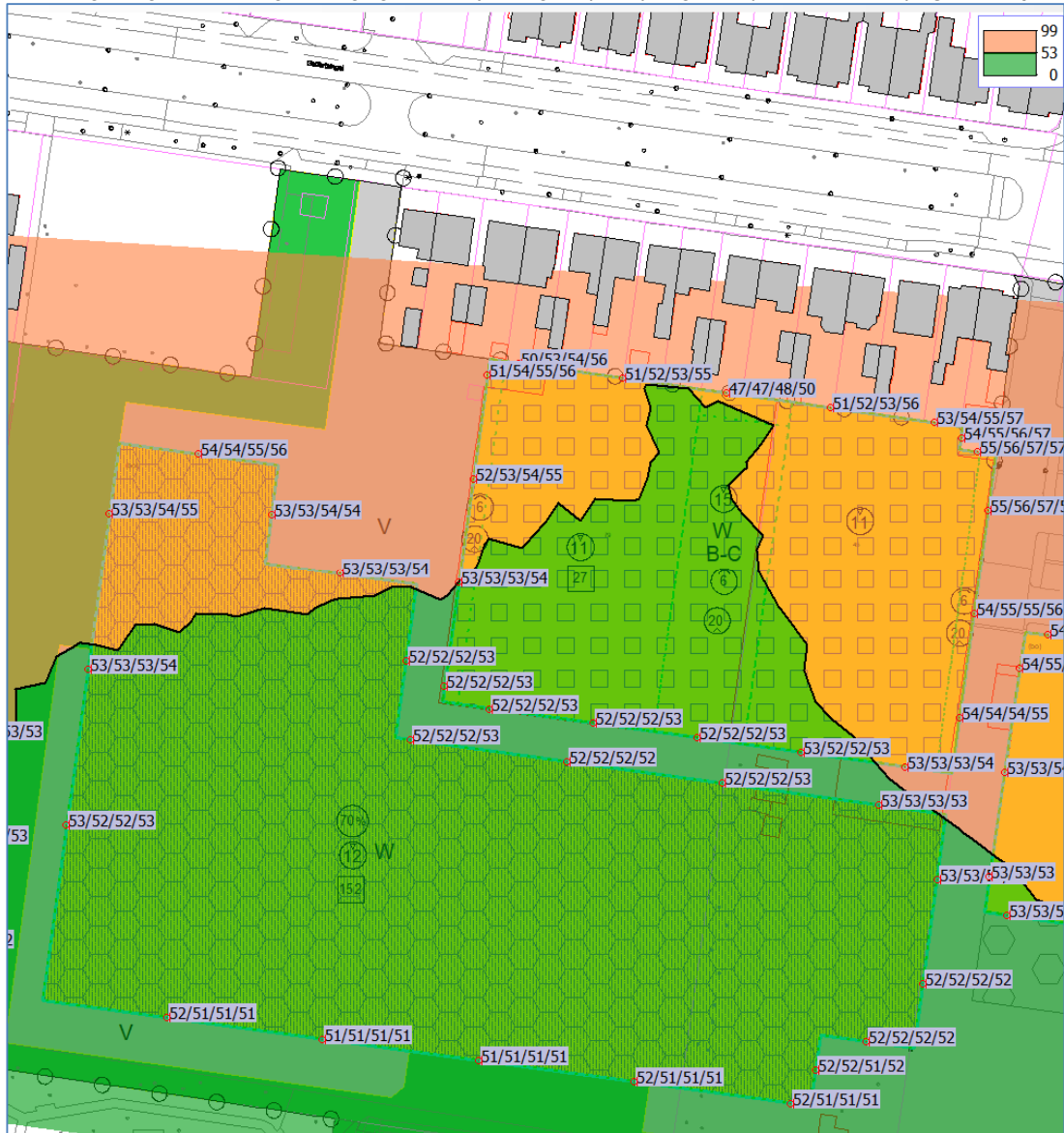
Afbeelding 2.2: geluidbelasting vanwege gemeentelijke wegen op het plangebied (Industriekwartier) bg/1°/ 2°/3°
