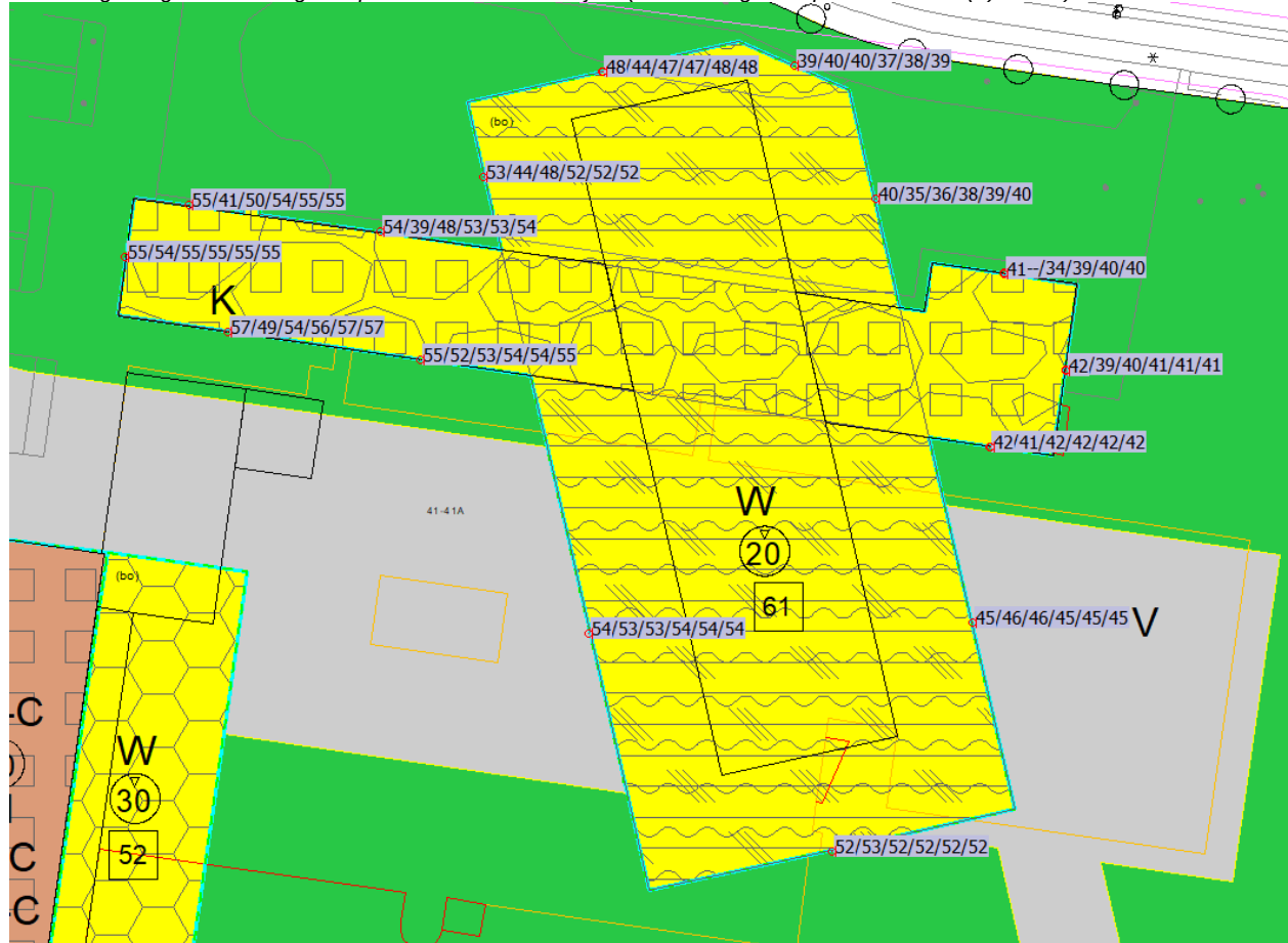
Afbeelding 3.8: geluidbelasting LAeq incidentele situatie 2x jaar (in voormalige drukpershal: 103 dB(A) House)
