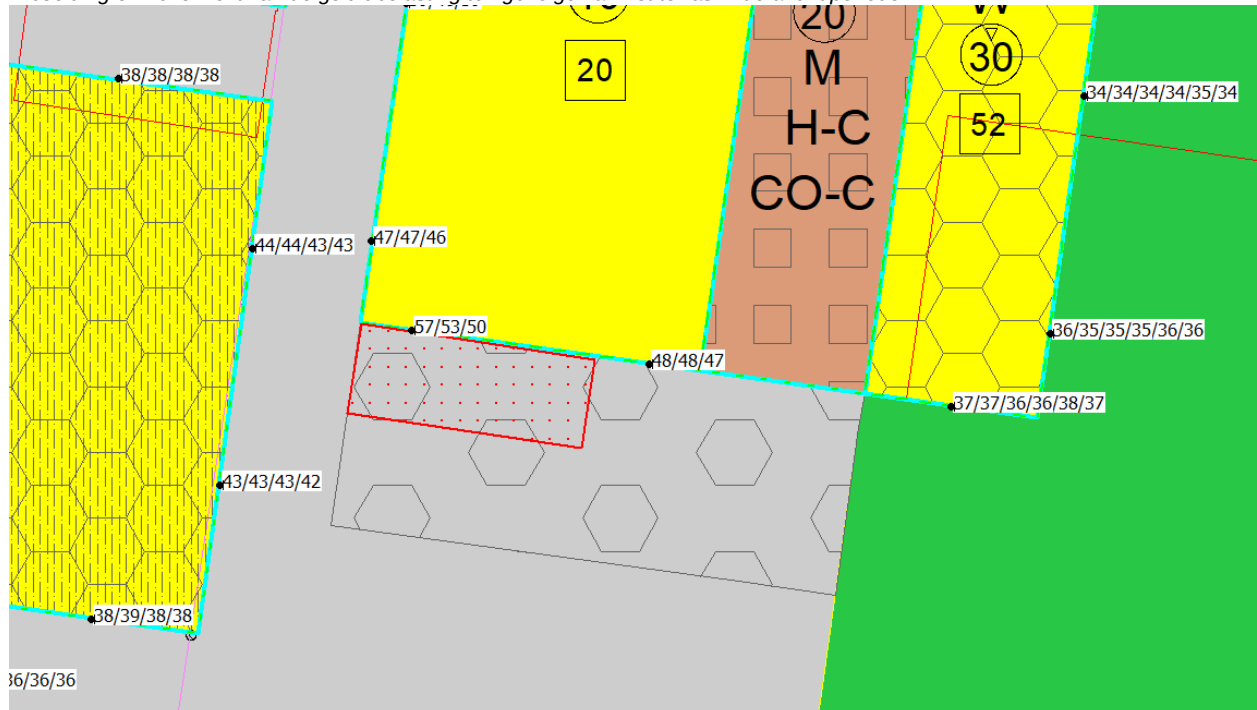
Afbeelding 3.2: overzicht van de geluidbelasting ten gevolge van het terras in de avondperiode.
