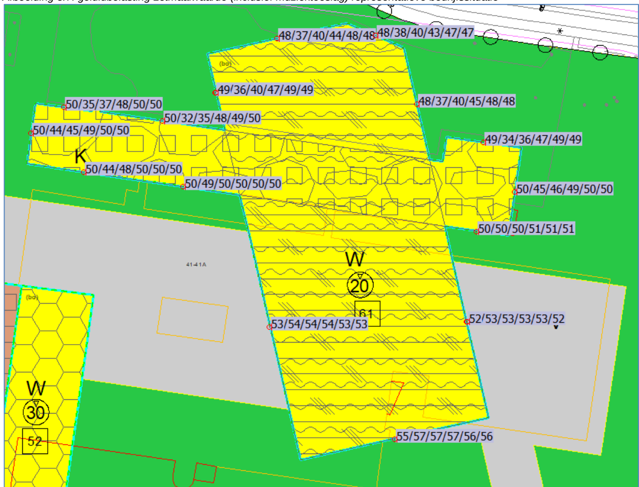
Afbeelding 3.7: geluidbelasting Letmaalwaarde (inclusief muziektoeslag) representatieve bedrijfssituatie
