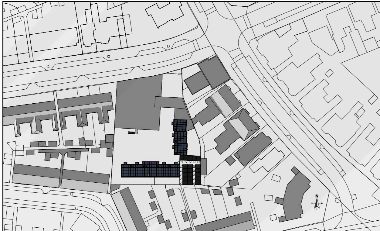
21 december 15:00uur
