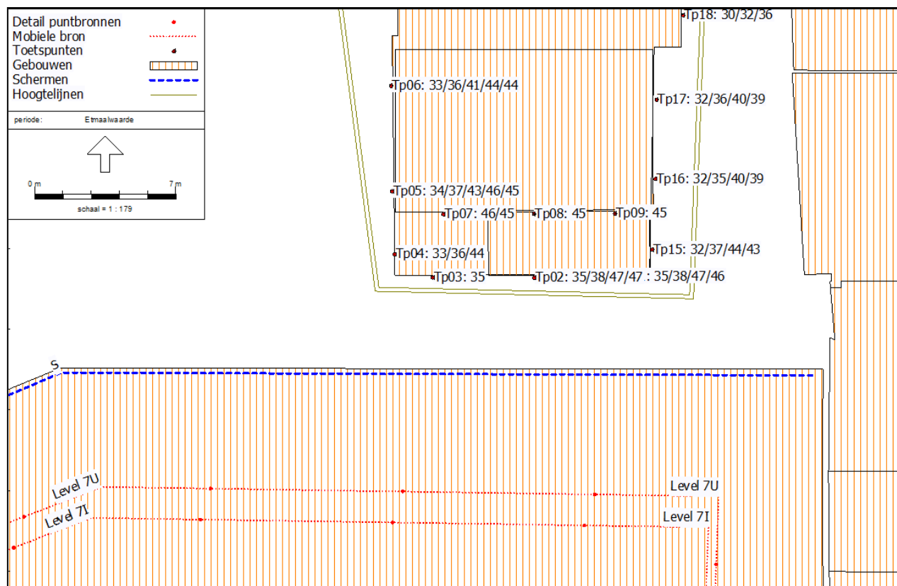
Afbeelding 6.1 Rekenresultaten L_{A,LT}
